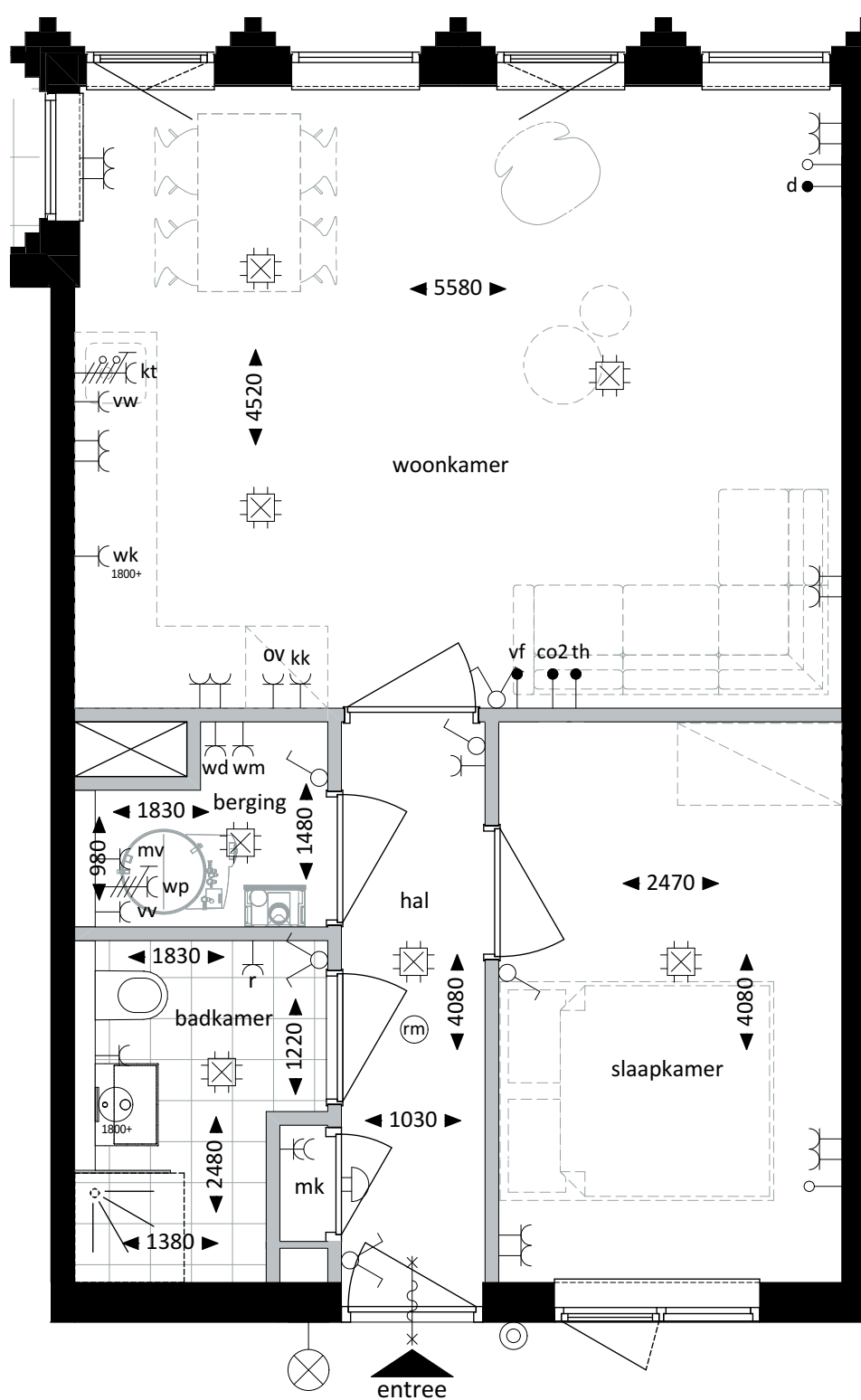
Plattegrond - 1:50
