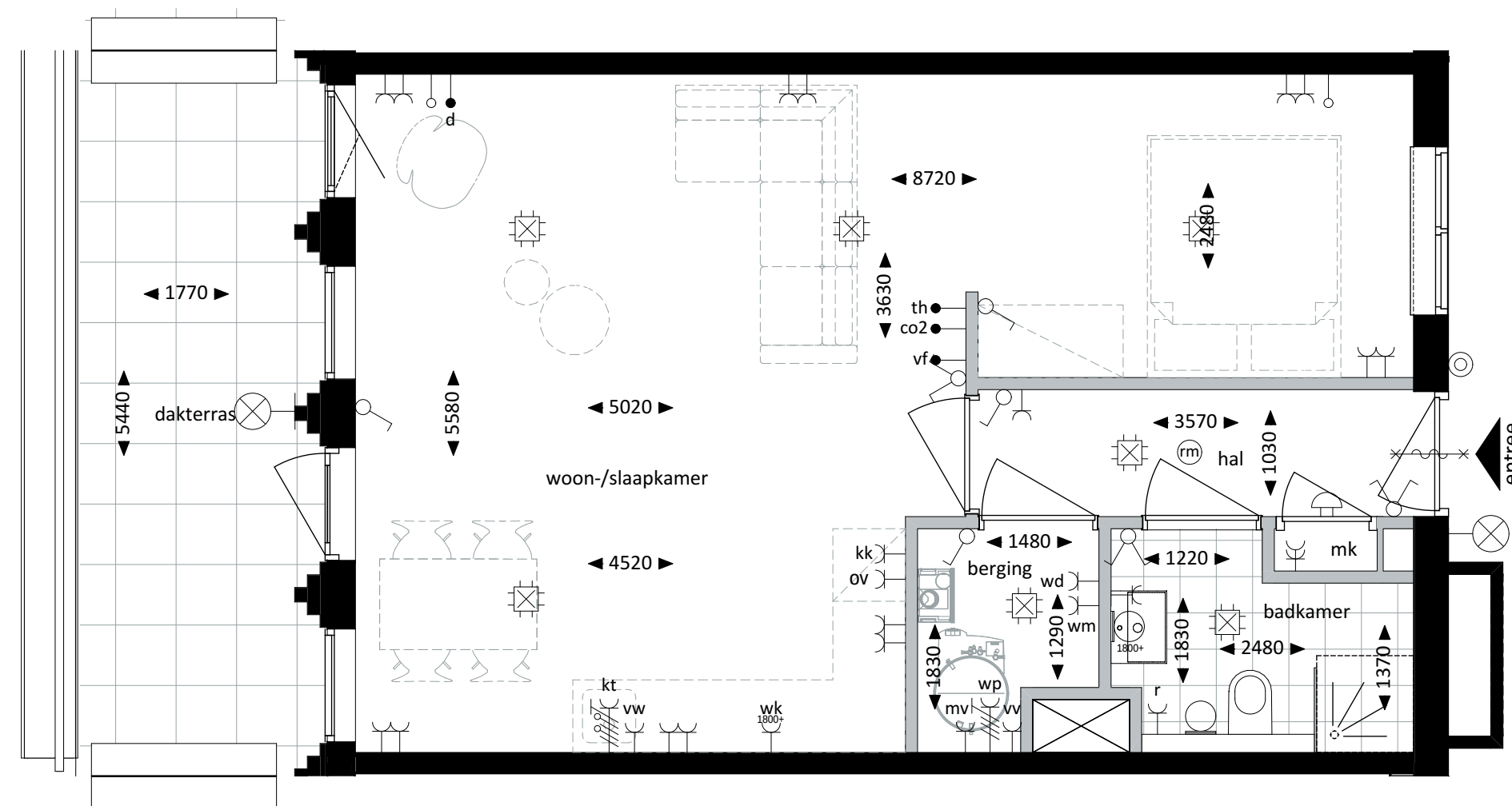
Plattegrond - 1:50
