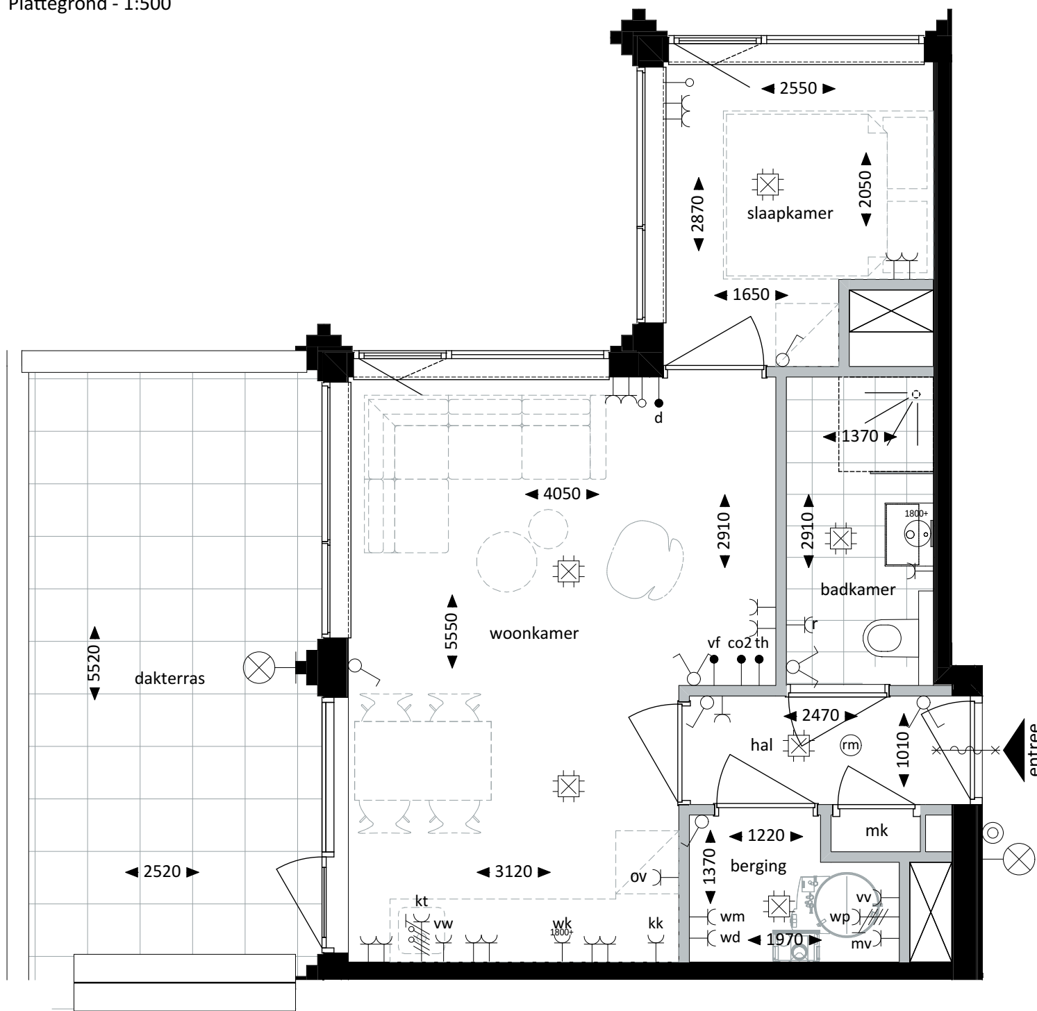
Plattegrond - 1:50
