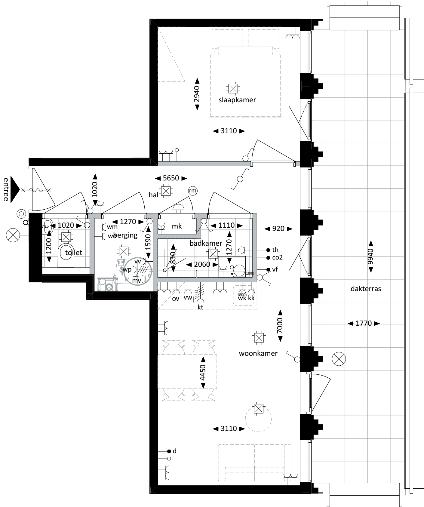
Plattegrond - 1:50
