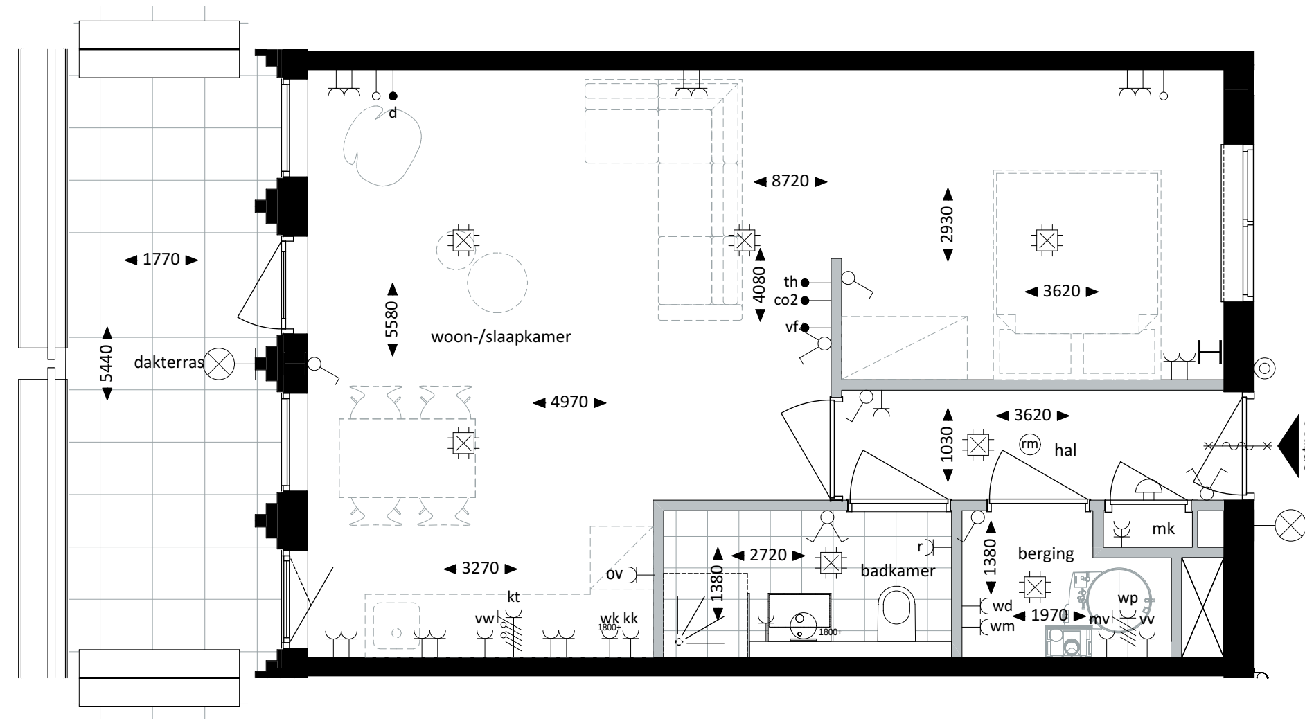
Plattegrond - 1:50
