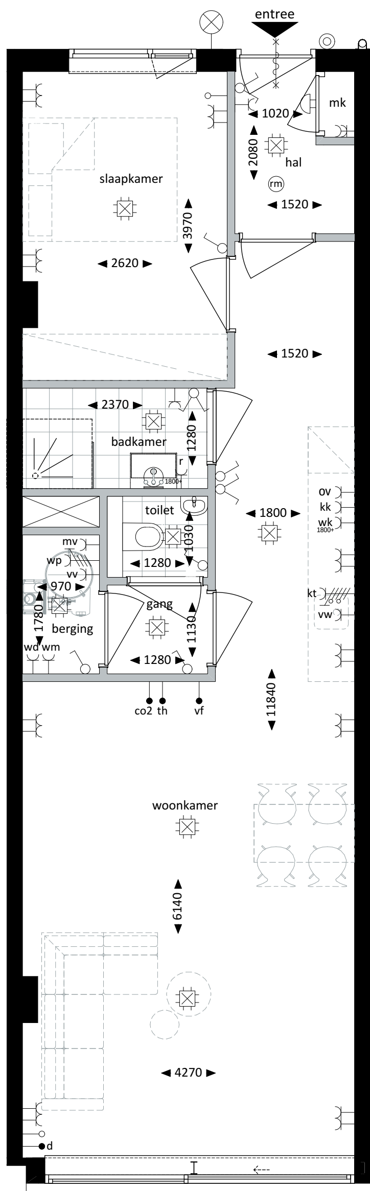
Plattegrond - 1:50
