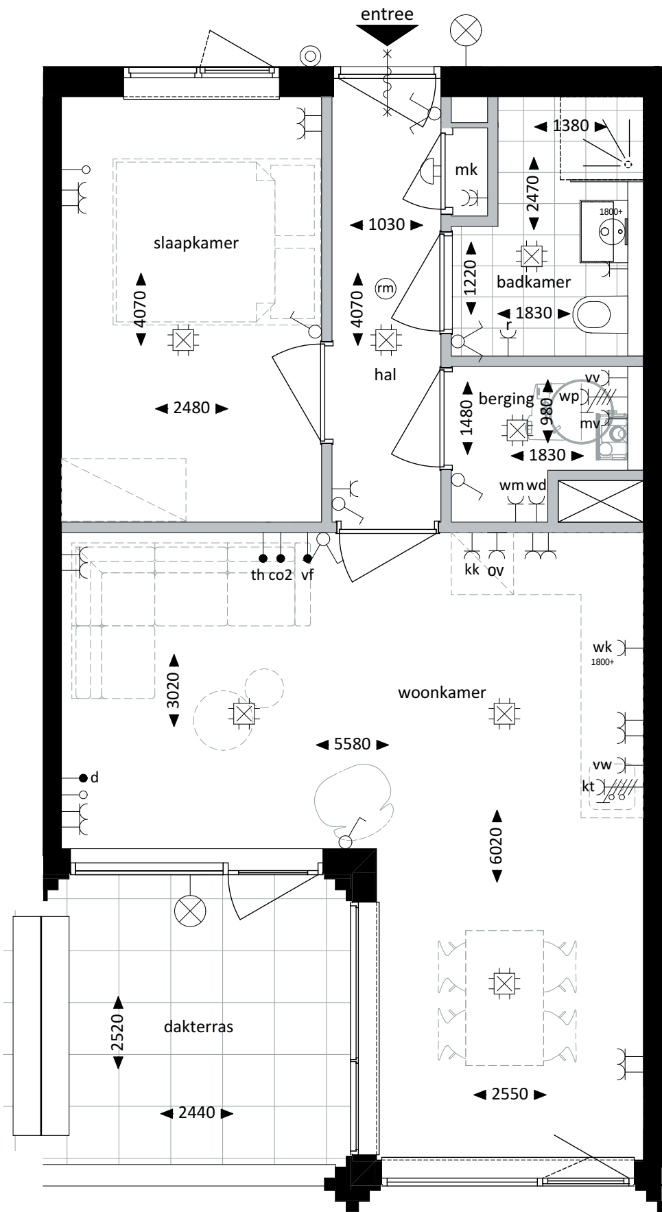
Plattegrond - 1:50
