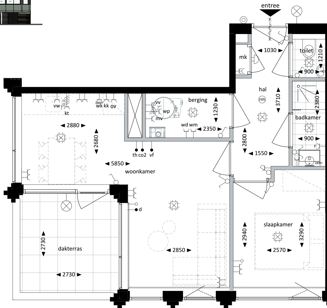
Plattegrond - 1:50
