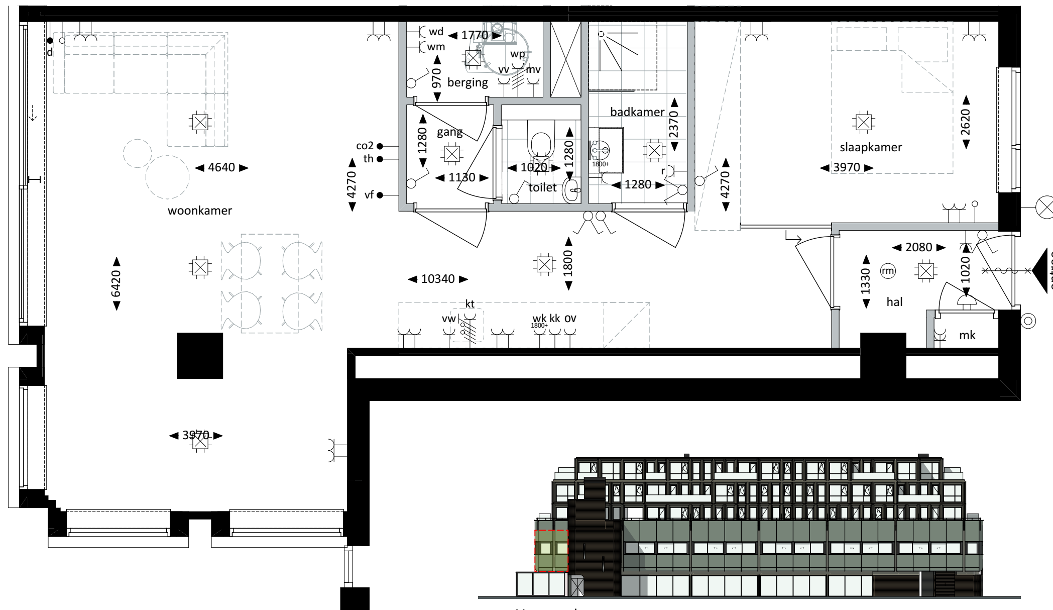
Plattegrond - 1:50
