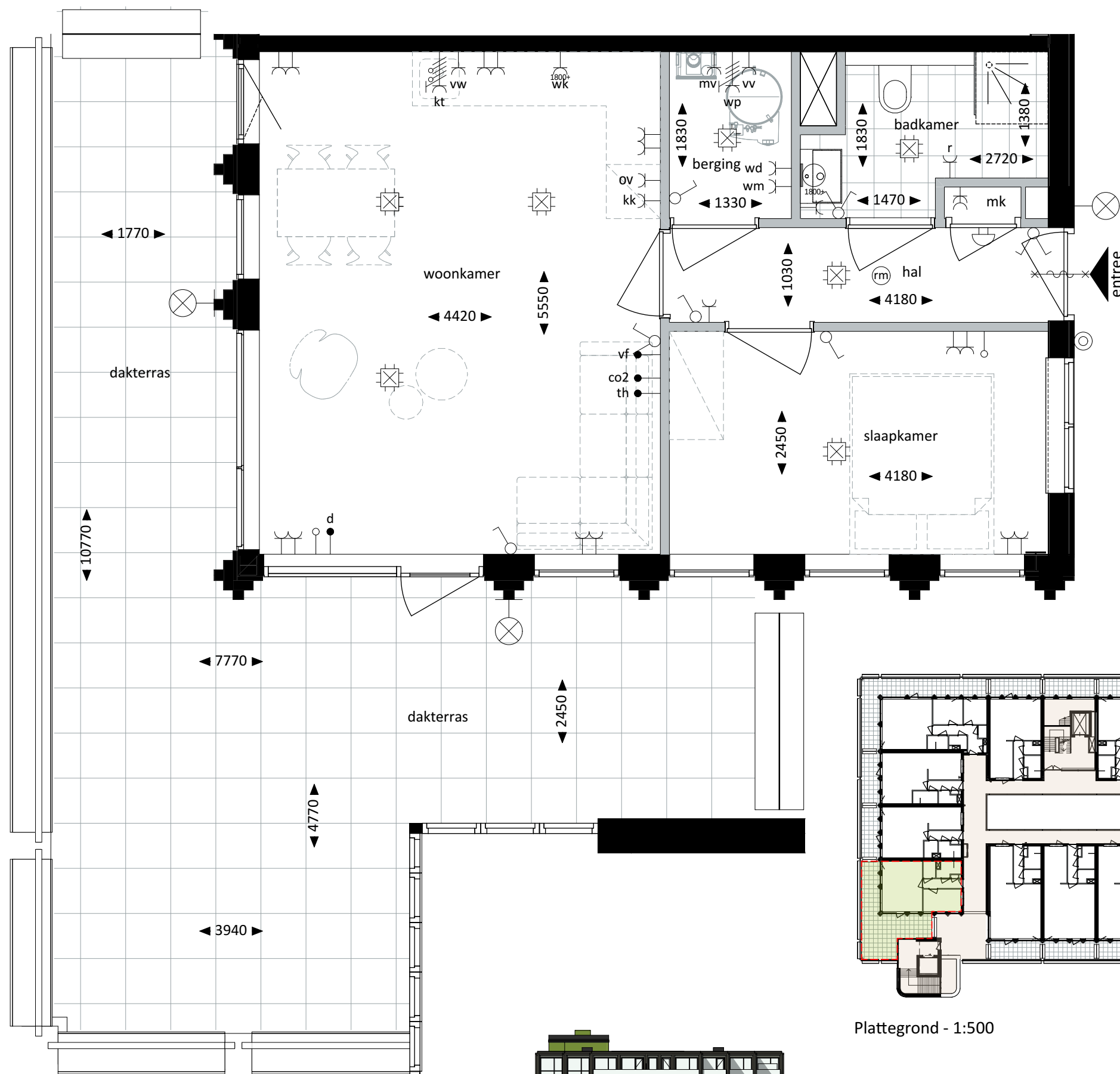
Plattegrond - 1:50
