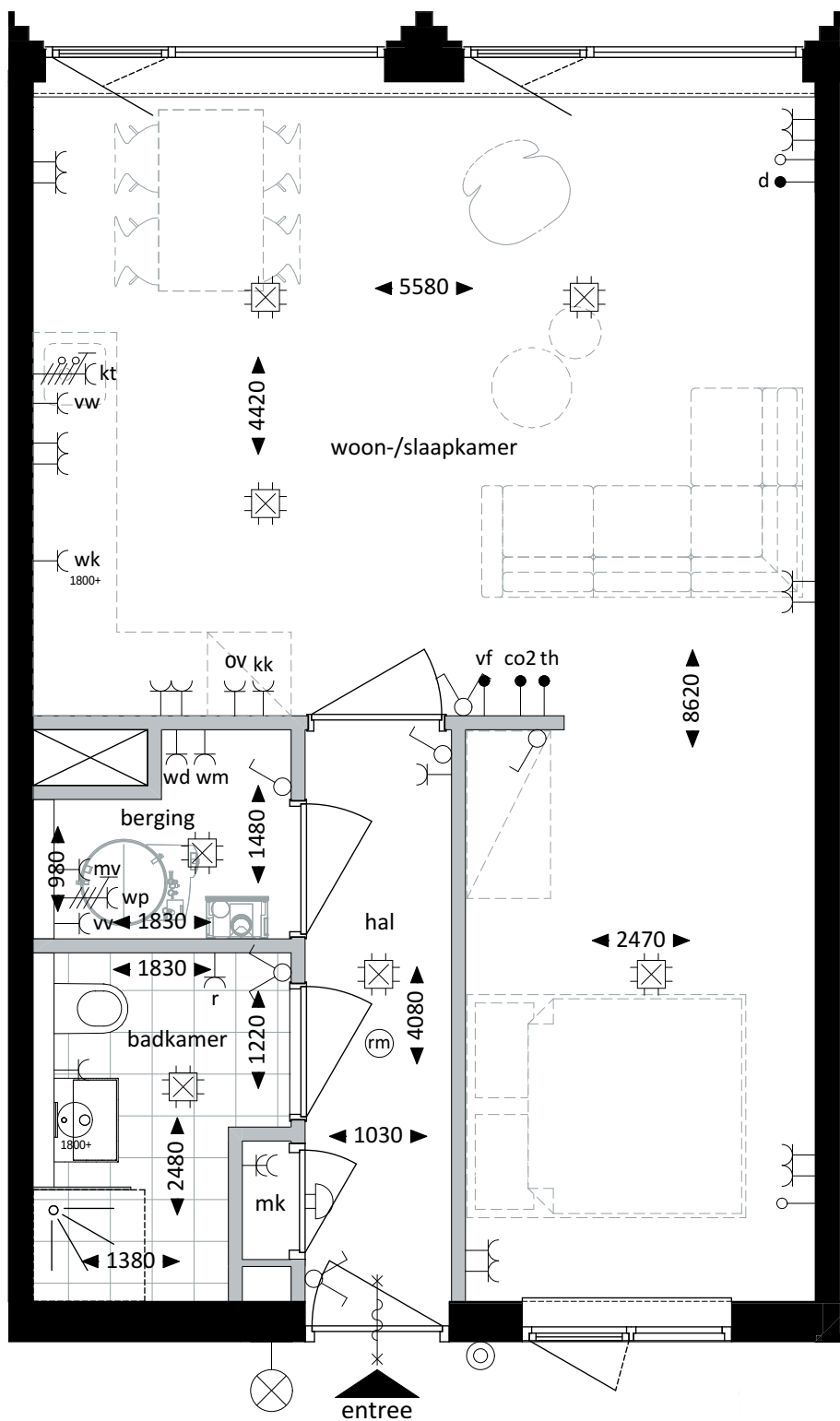
Plattegrond - 1:50
