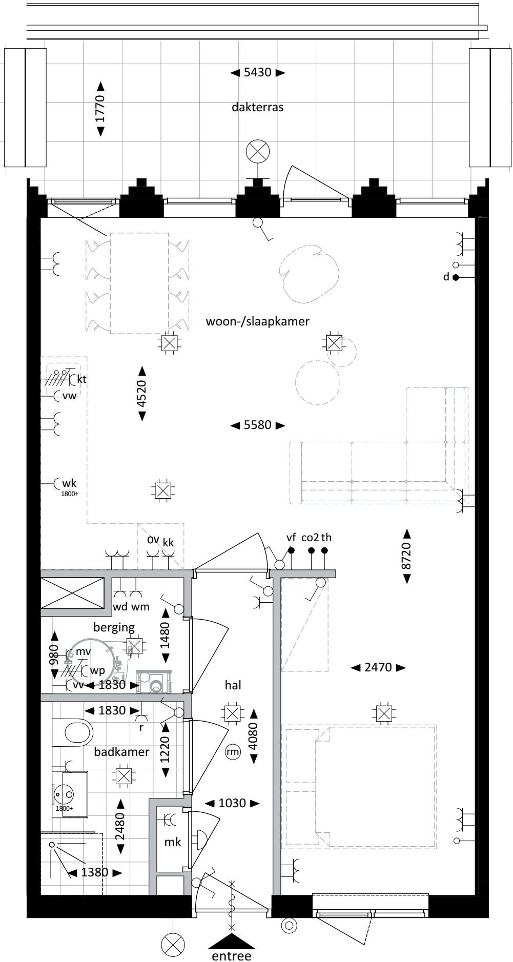
Plattegrond - 1:50
