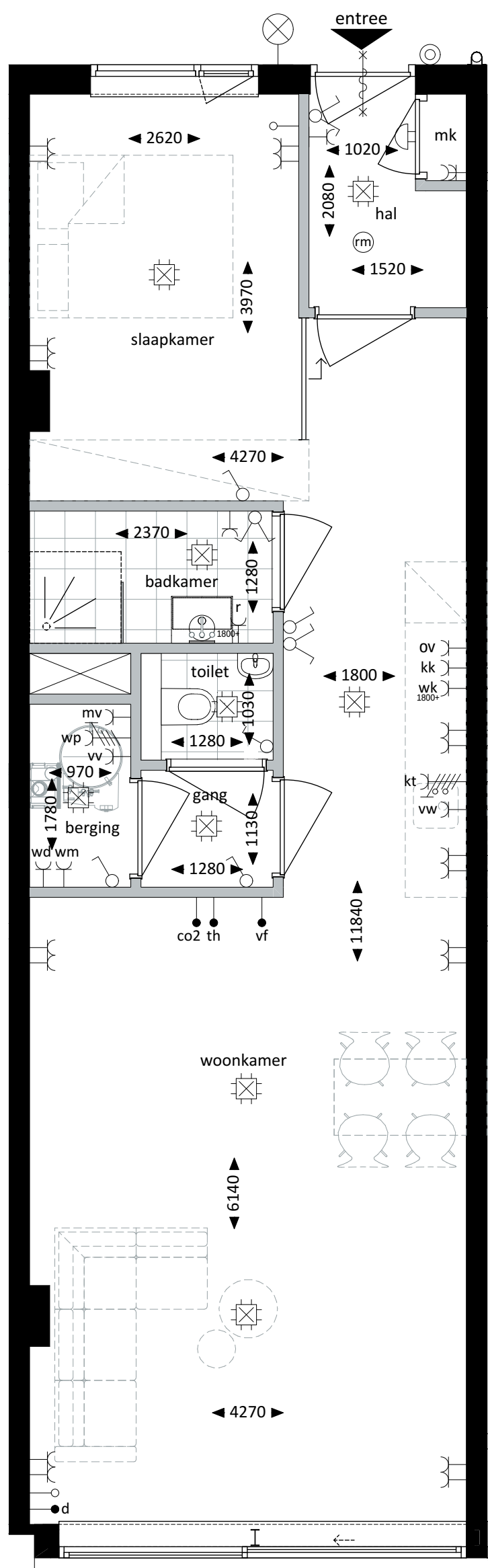
Plattegrond - 1:50
