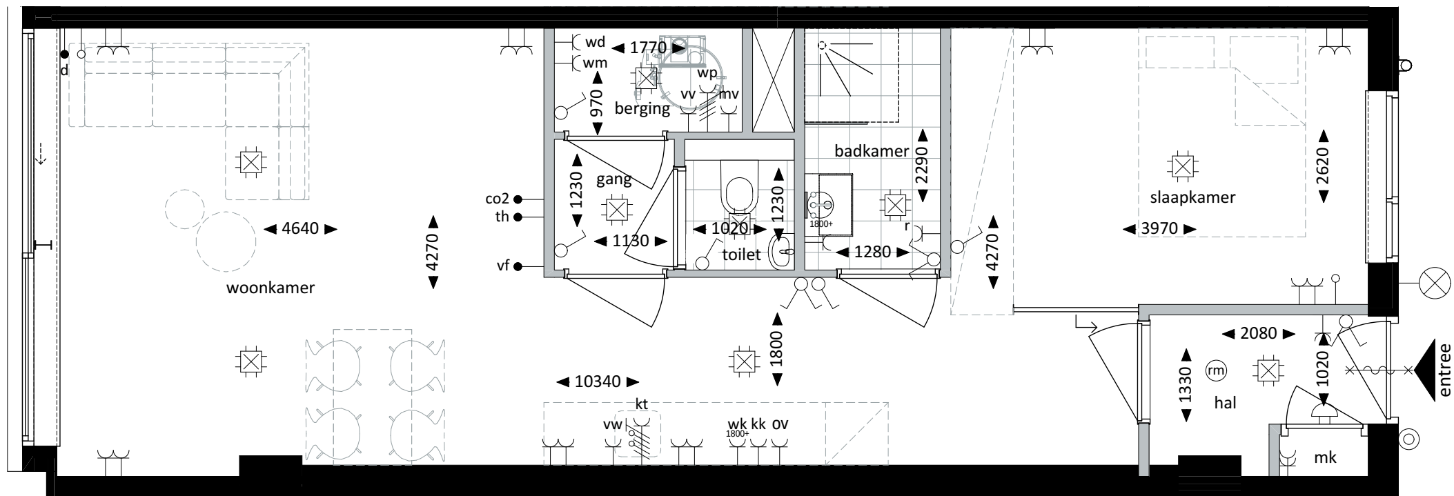
Plattegrond - 1:50
