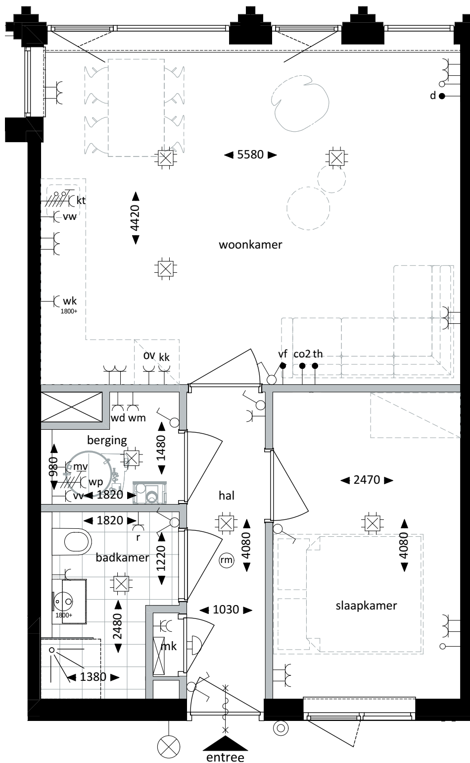
Plattegrond - 1:50
