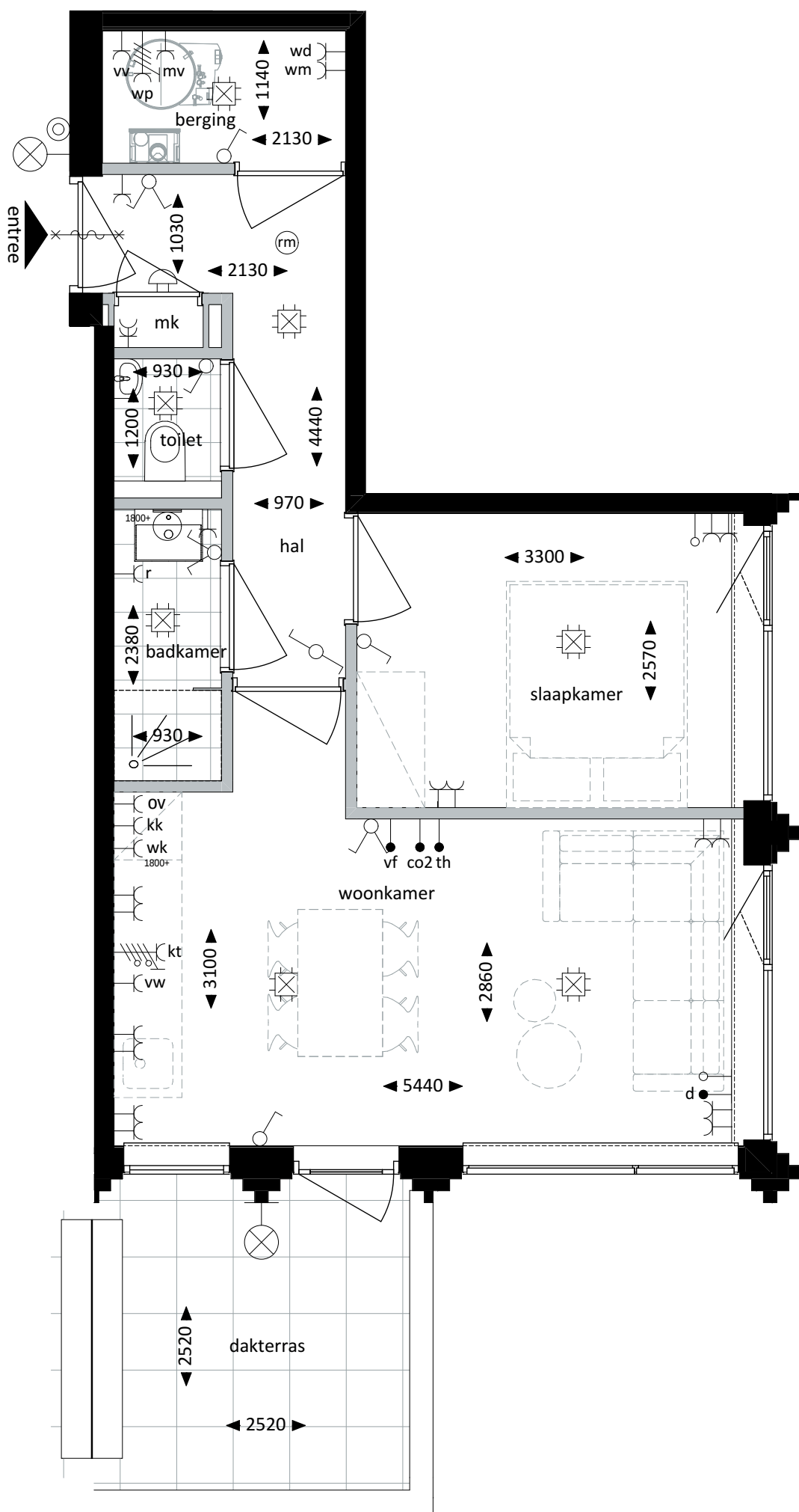
Plattegrond - 1:50
