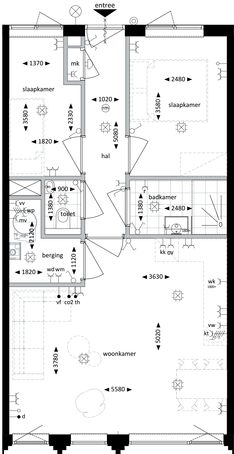
Plattegrond - 1:50
