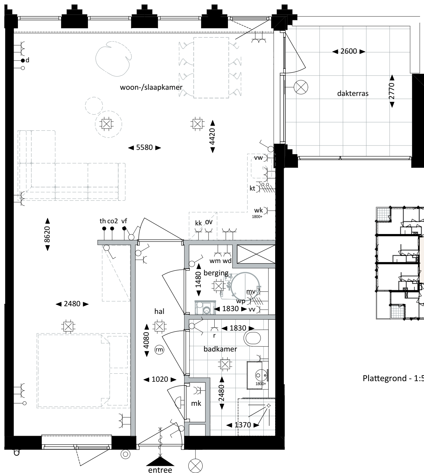
Plattegrond - 1:50
