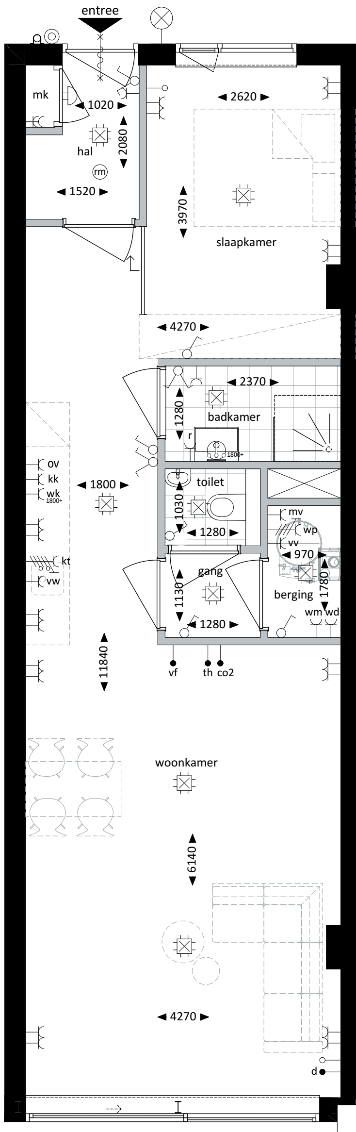
Plattegrond - 1:50
