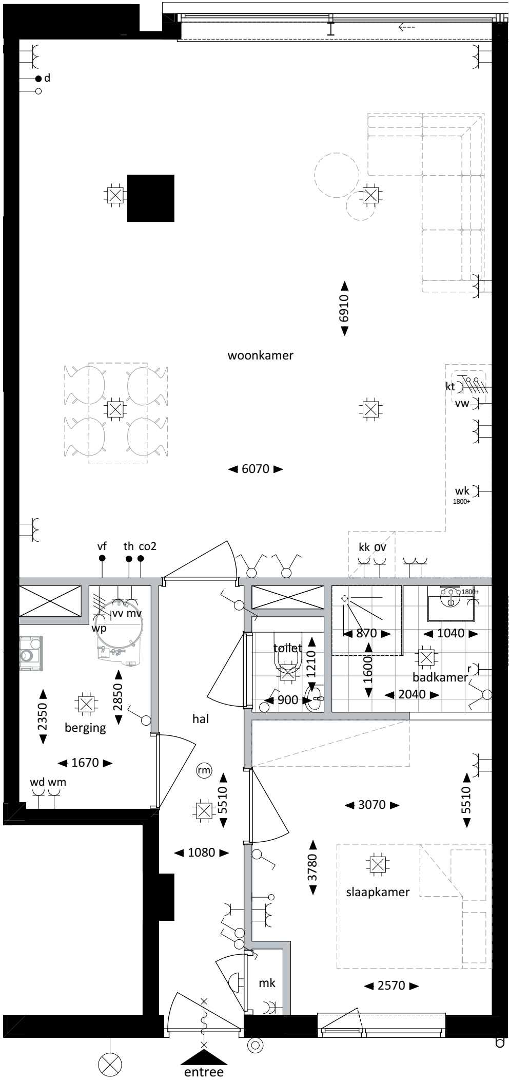
Plattegrond - 1:50
