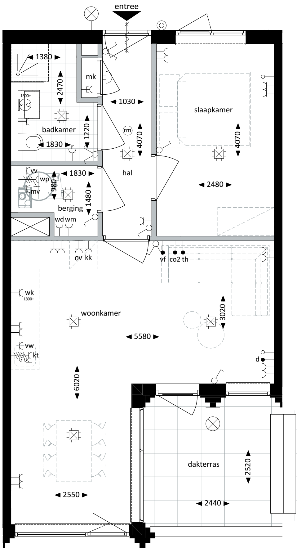
Plattegrond - 1:50
