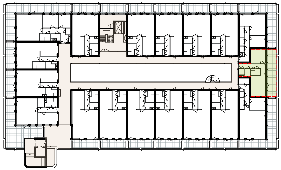
Plattegrond - 1:500
