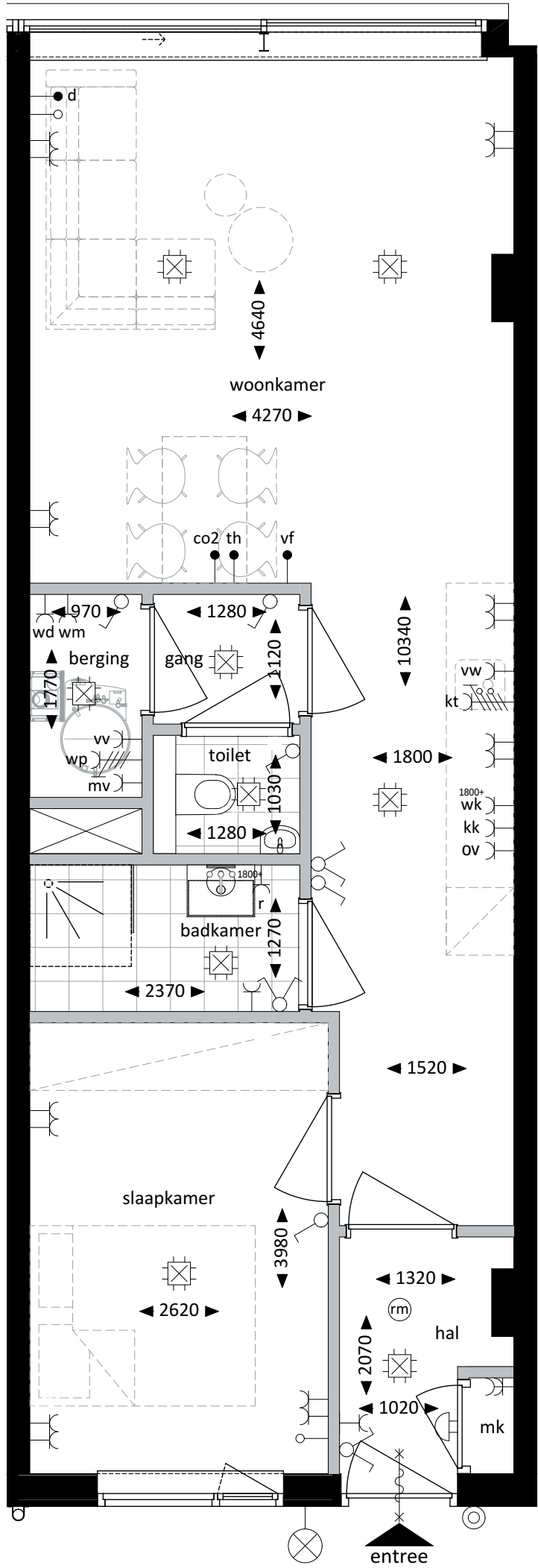
Plattegrond - 1:50
