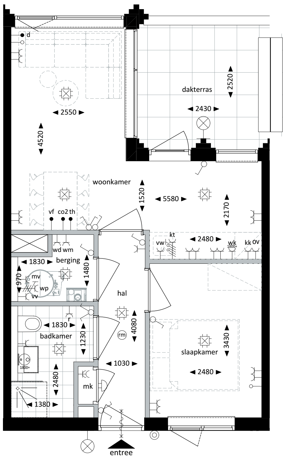
Plattegrond - 1:50
