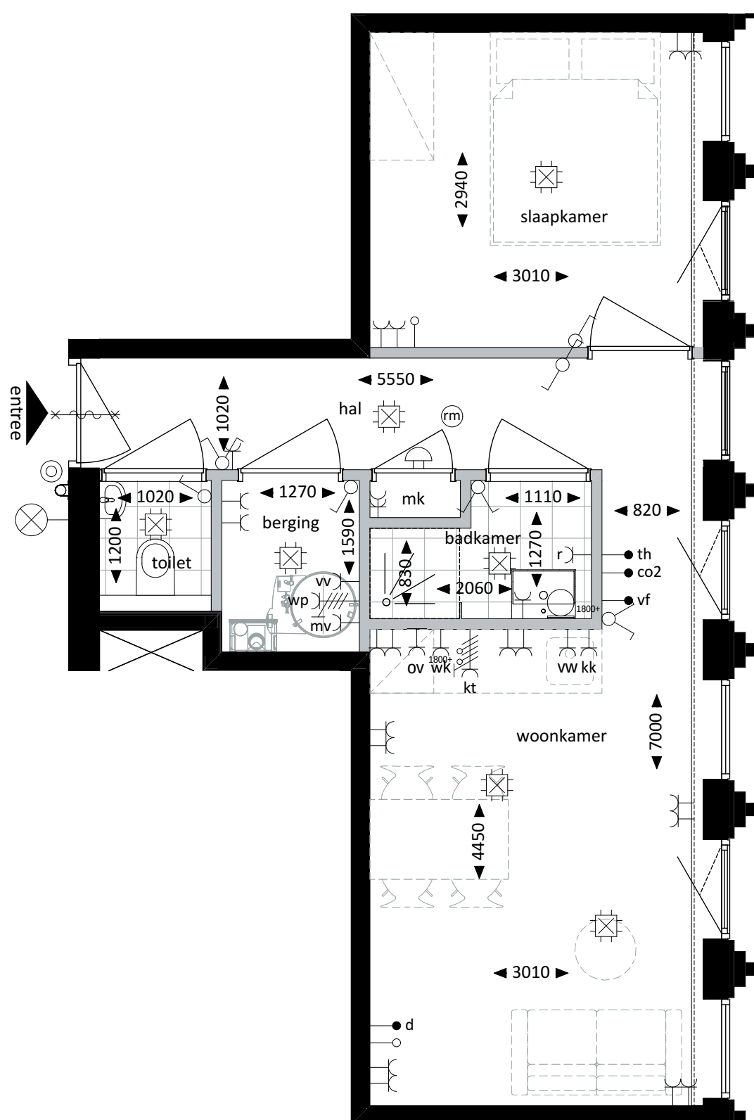
Plattegrond - 1:50
