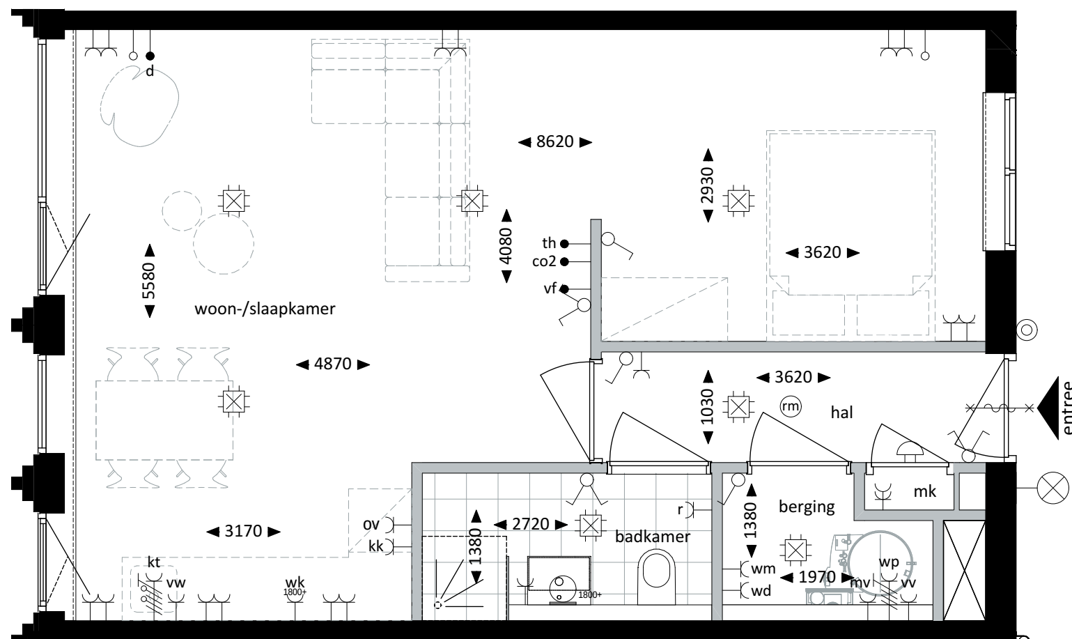
Plattegrond - 1:50
