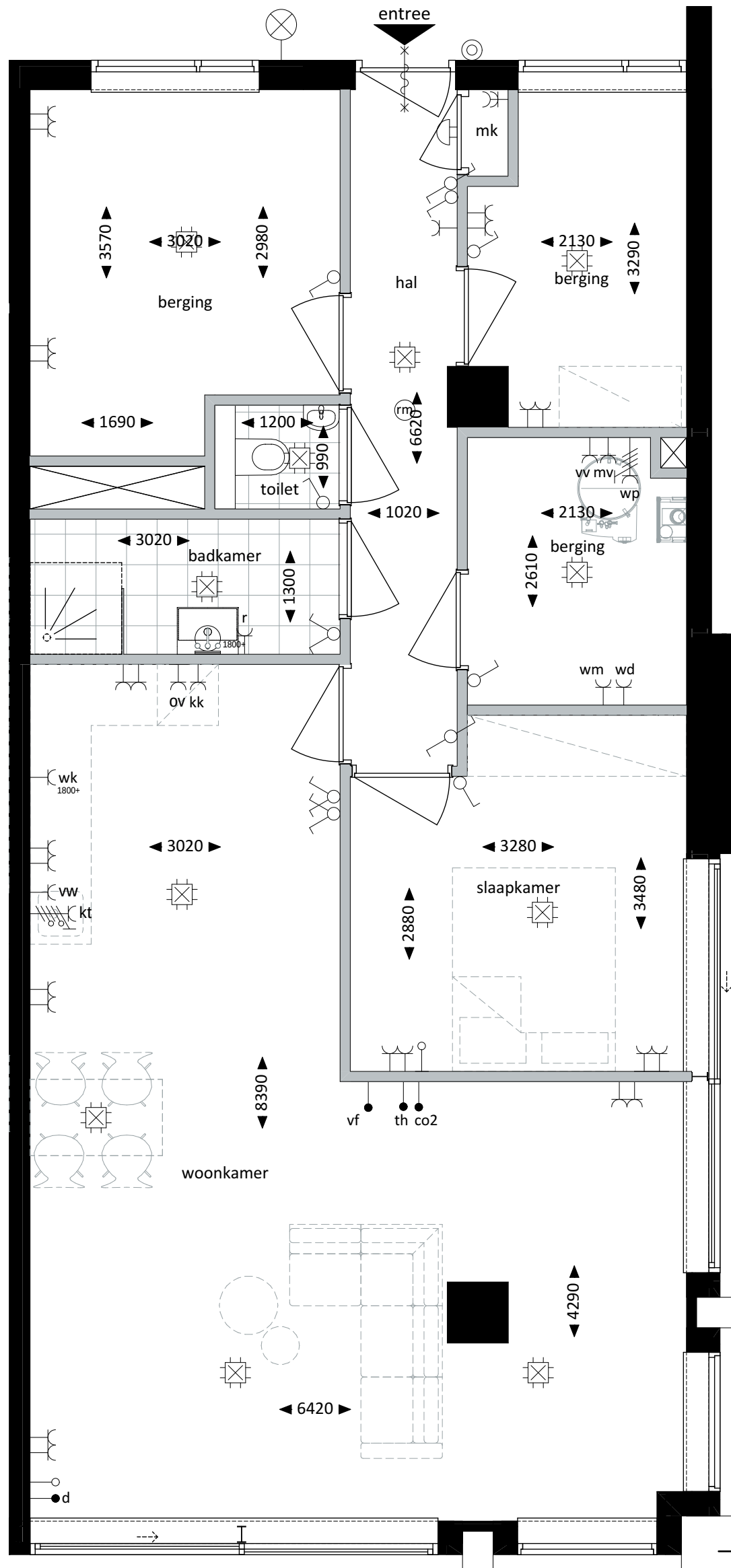
Plattegrond - 1:50
