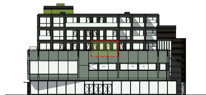
Linker zijgevel
