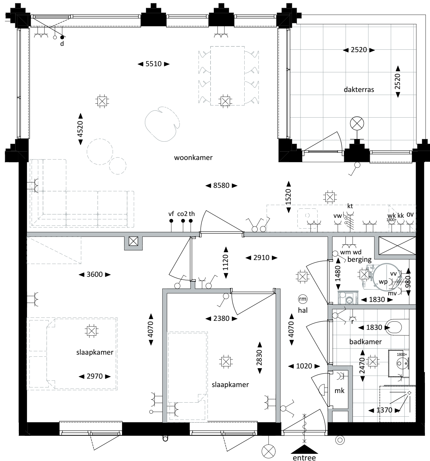
Plattegrond - 1:50
