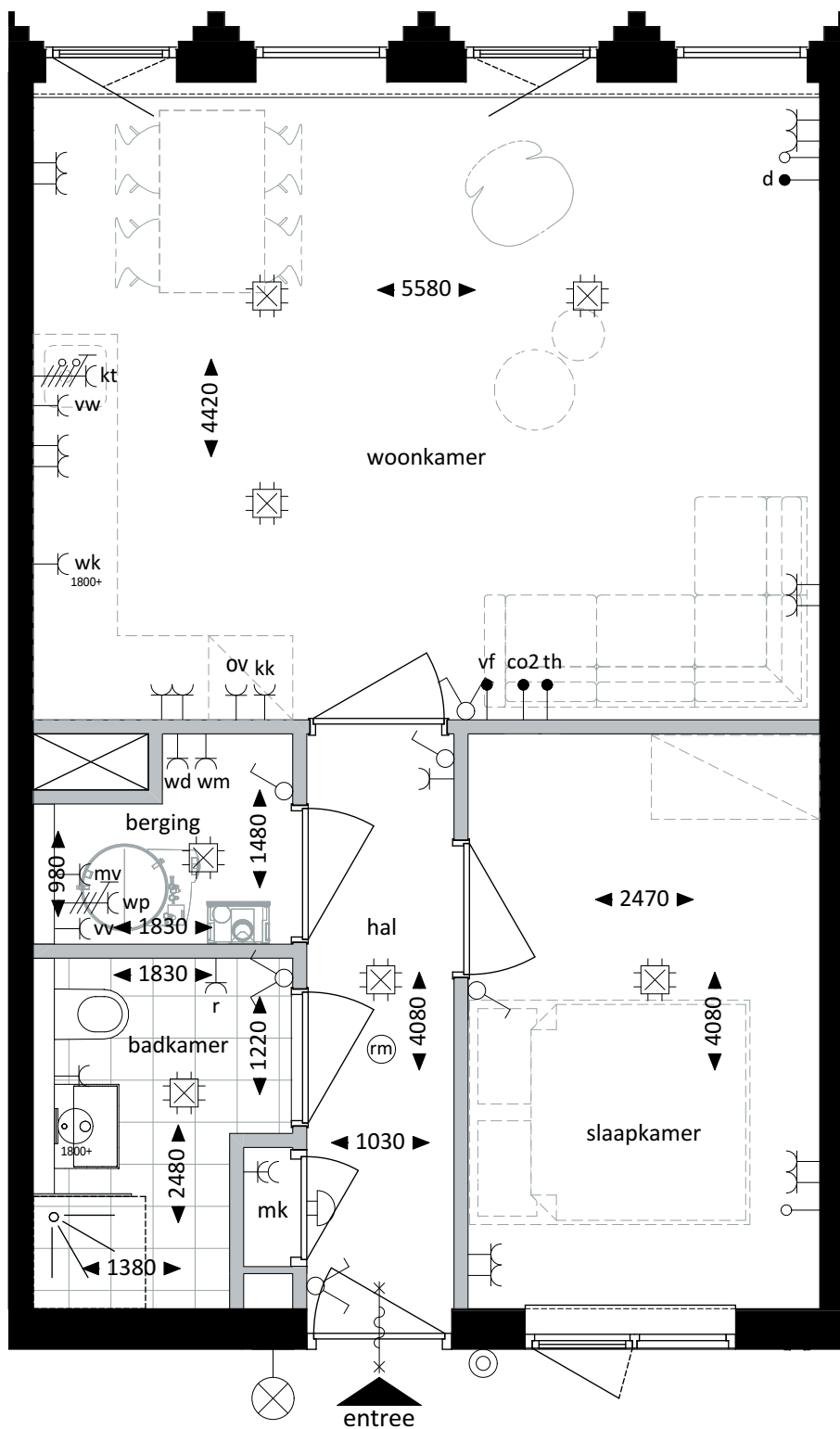
Plattegrond - 1:50
