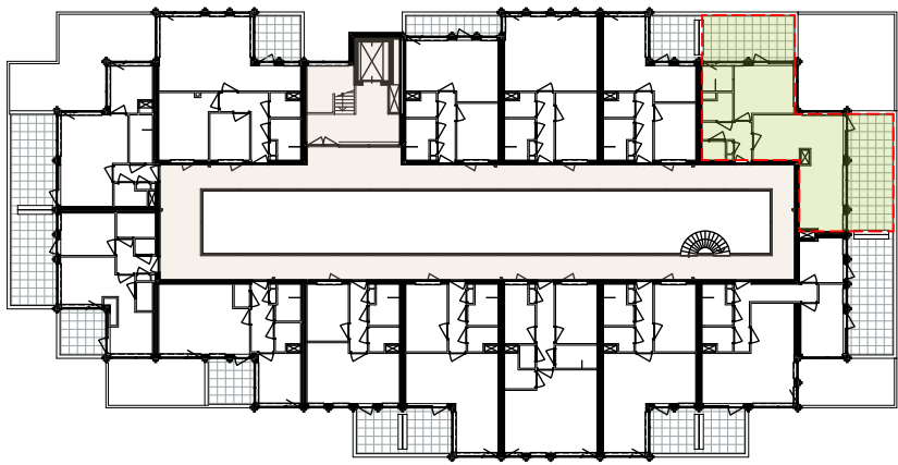
Plattegrond - 1:500
