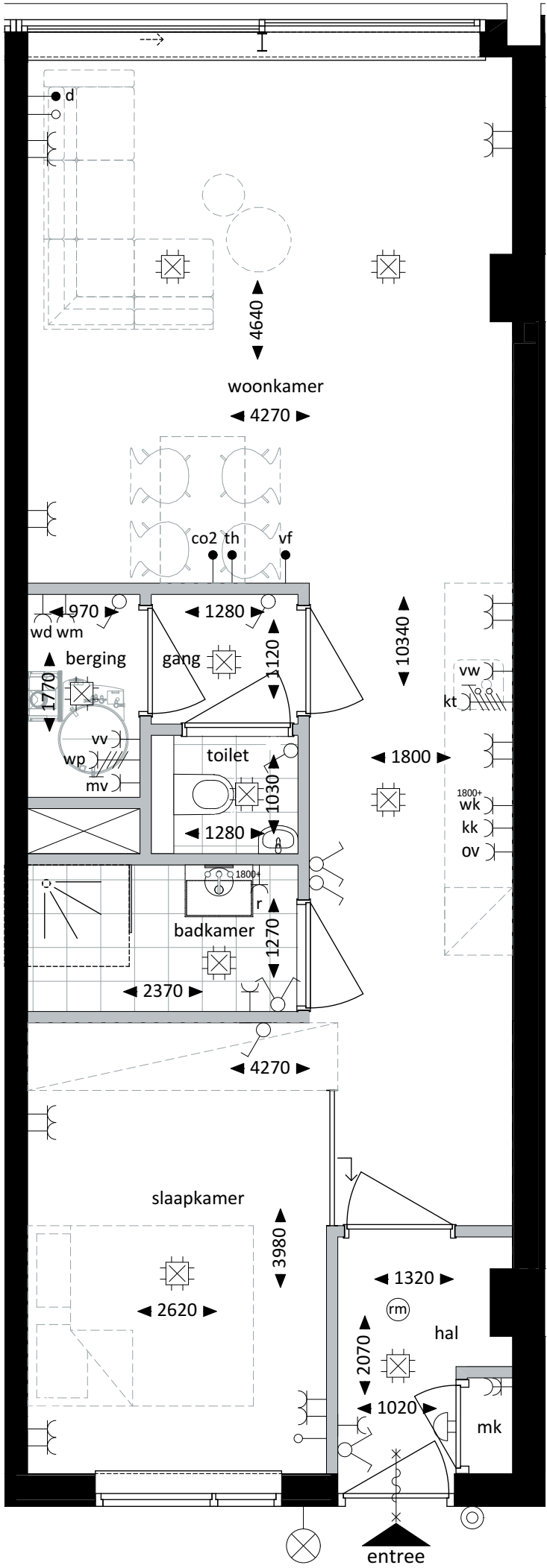
Plattegrond - 1:50
