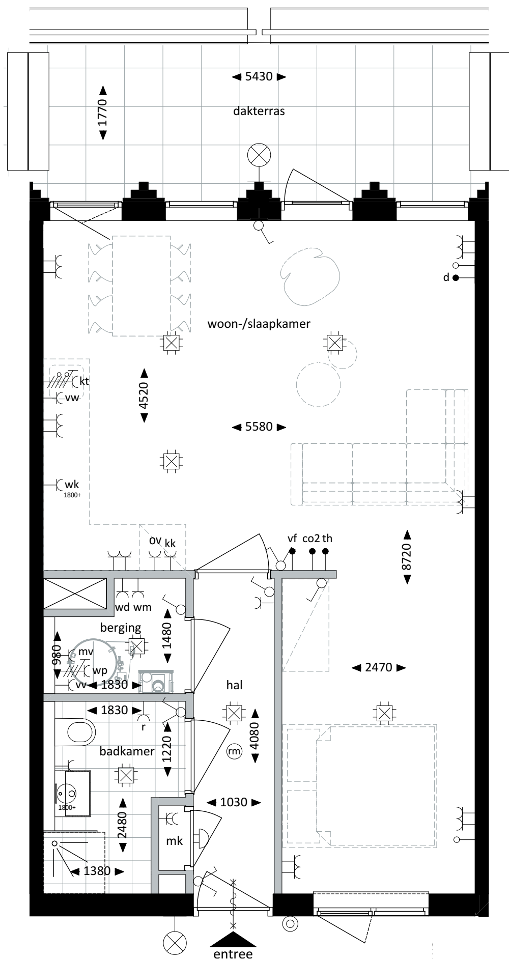
Plattegrond - 1:50
