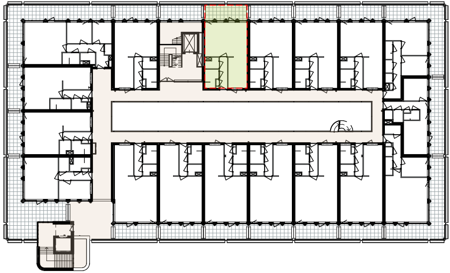
Plattegrond - 1:500
