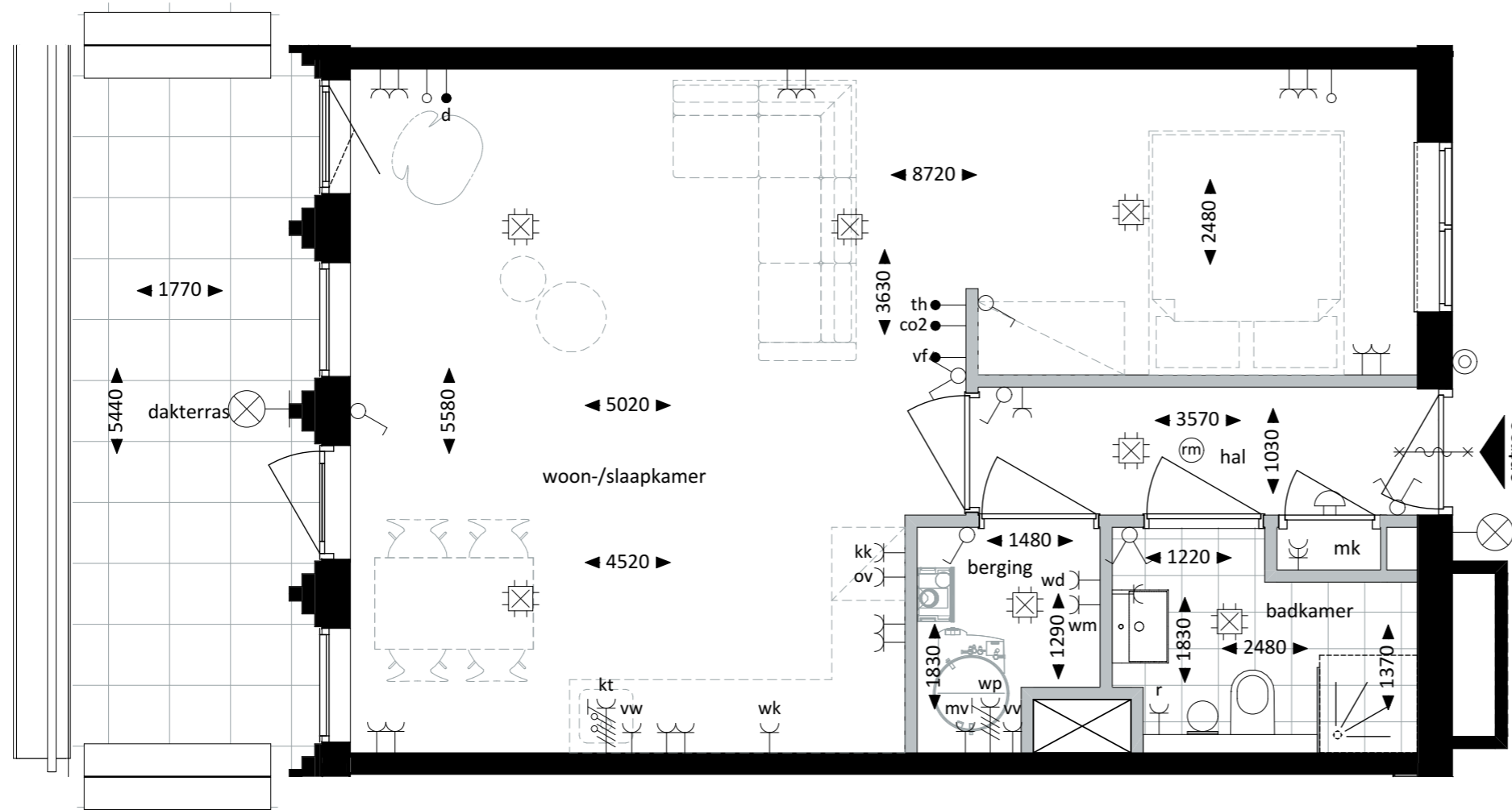
Plattegrond - 1:50
