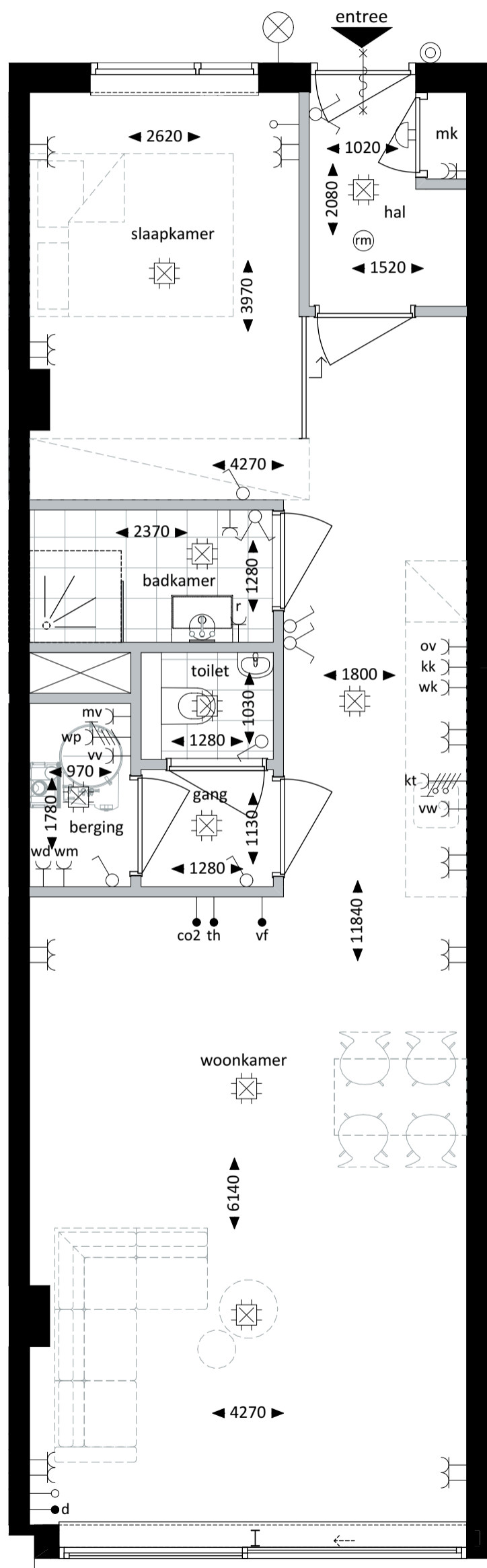
Plattegrond - 1:50
