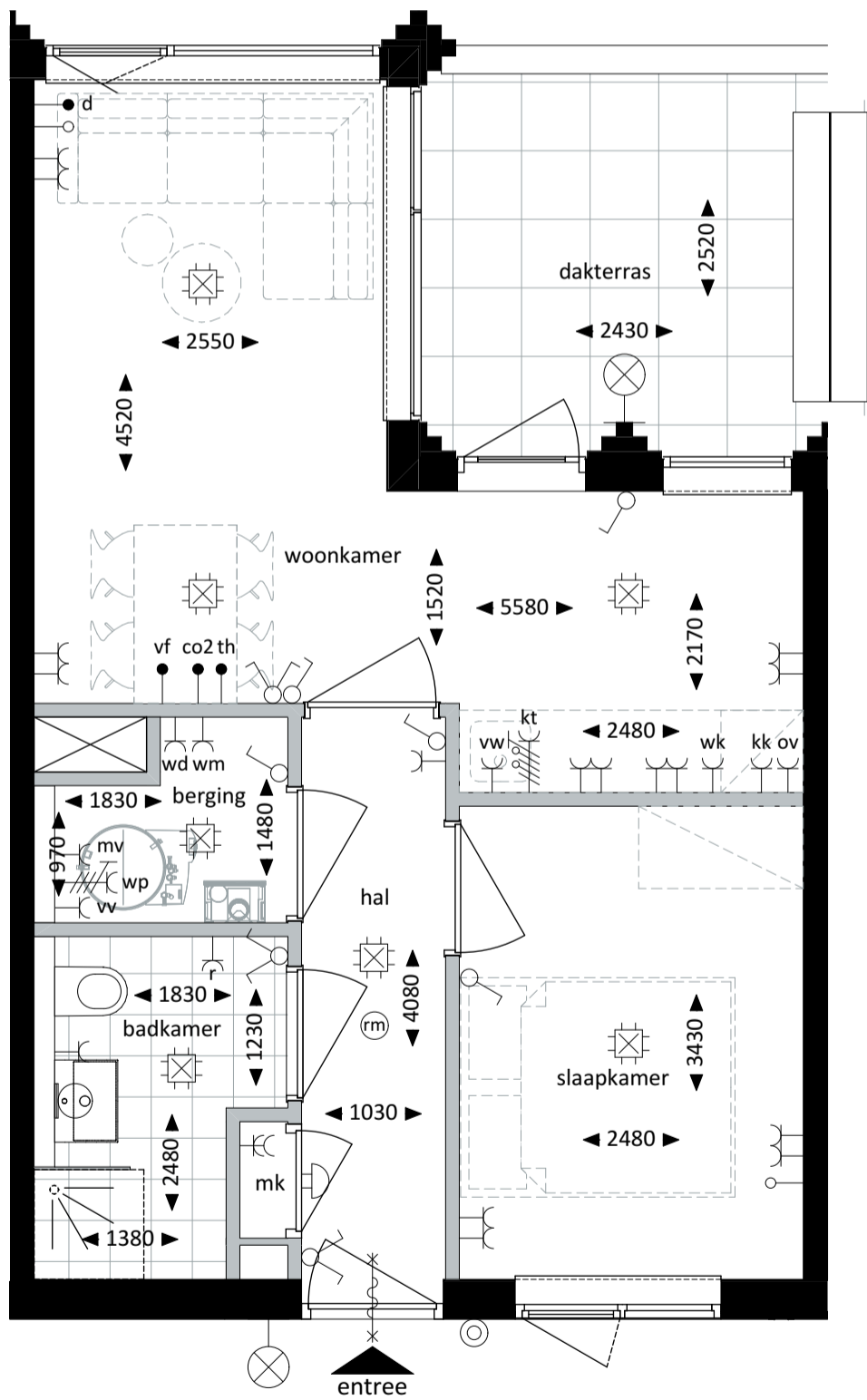
Plattegrond - 1:50
