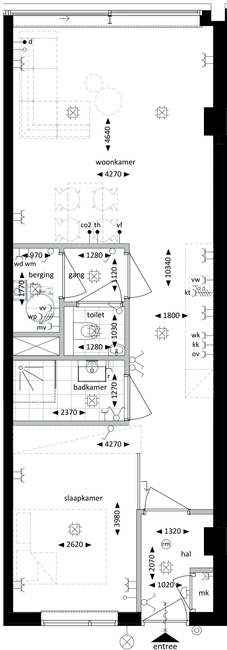
Plattegrond - 1:50
