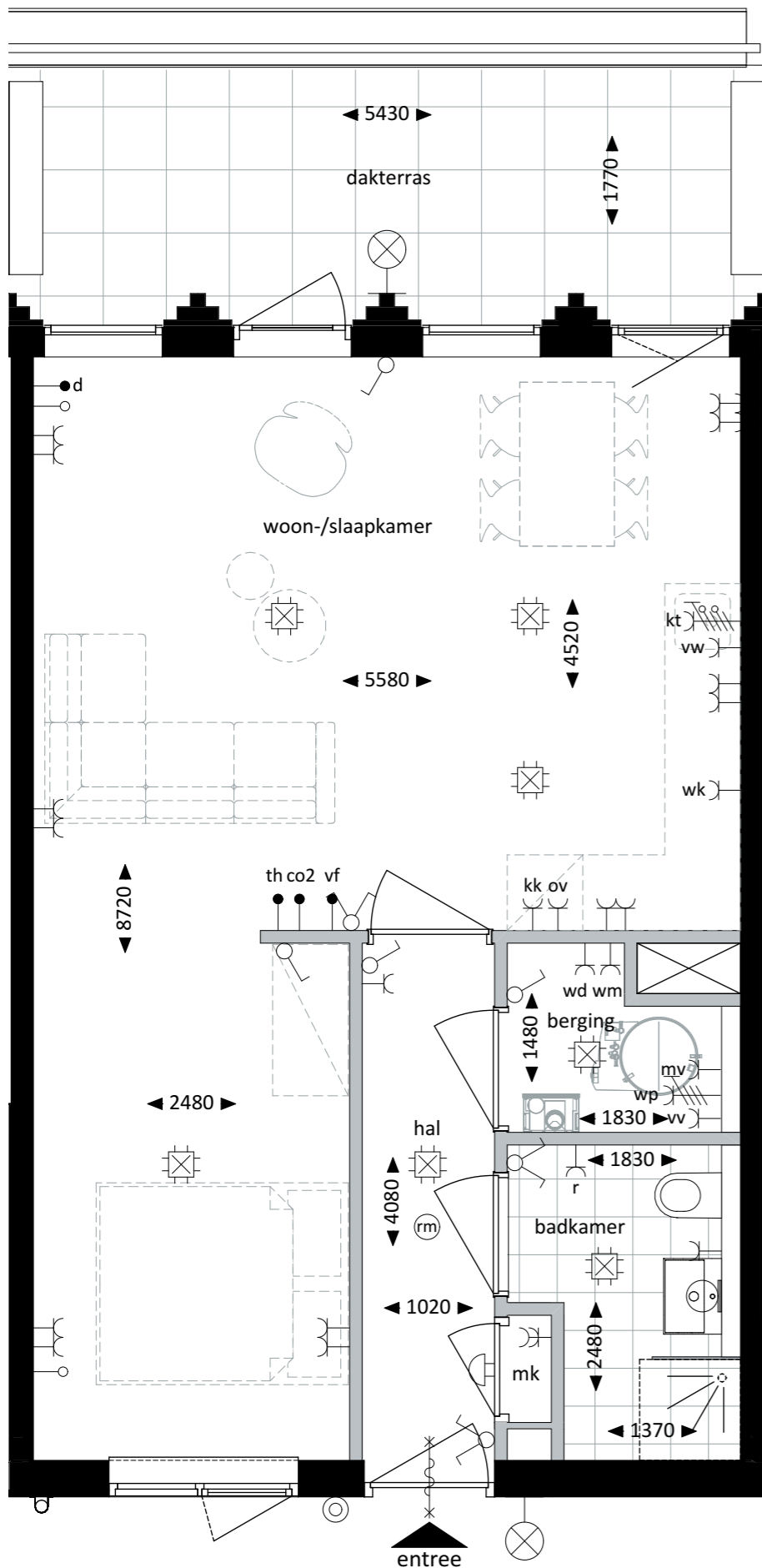
Plattegrond - 1:50
