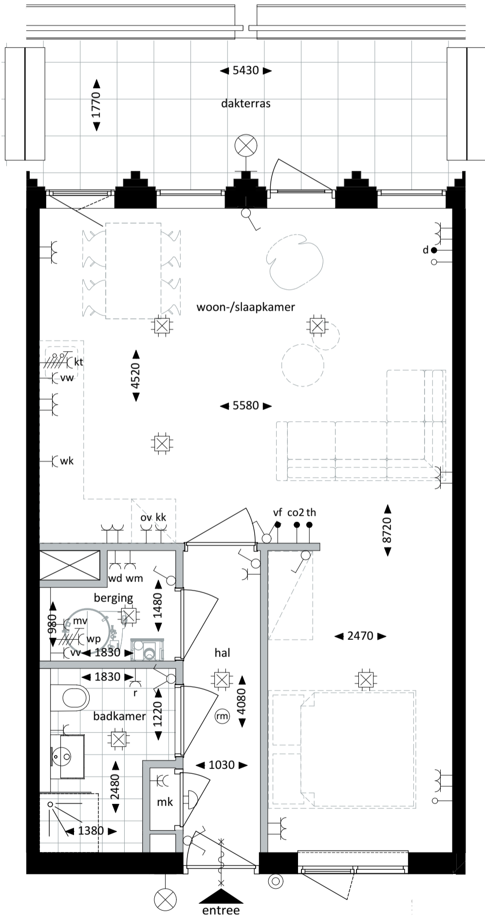
Plattegrond - 1:50
