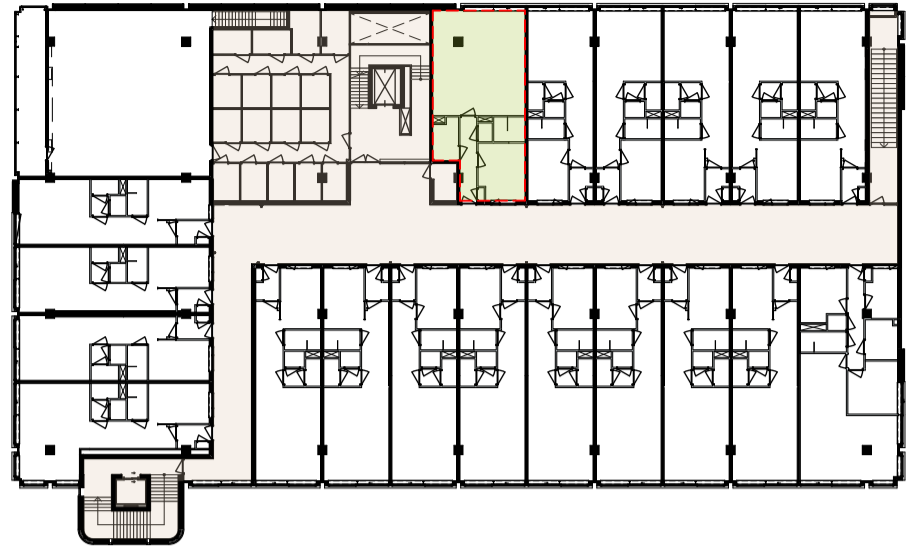
Plattegrond - 1:500
