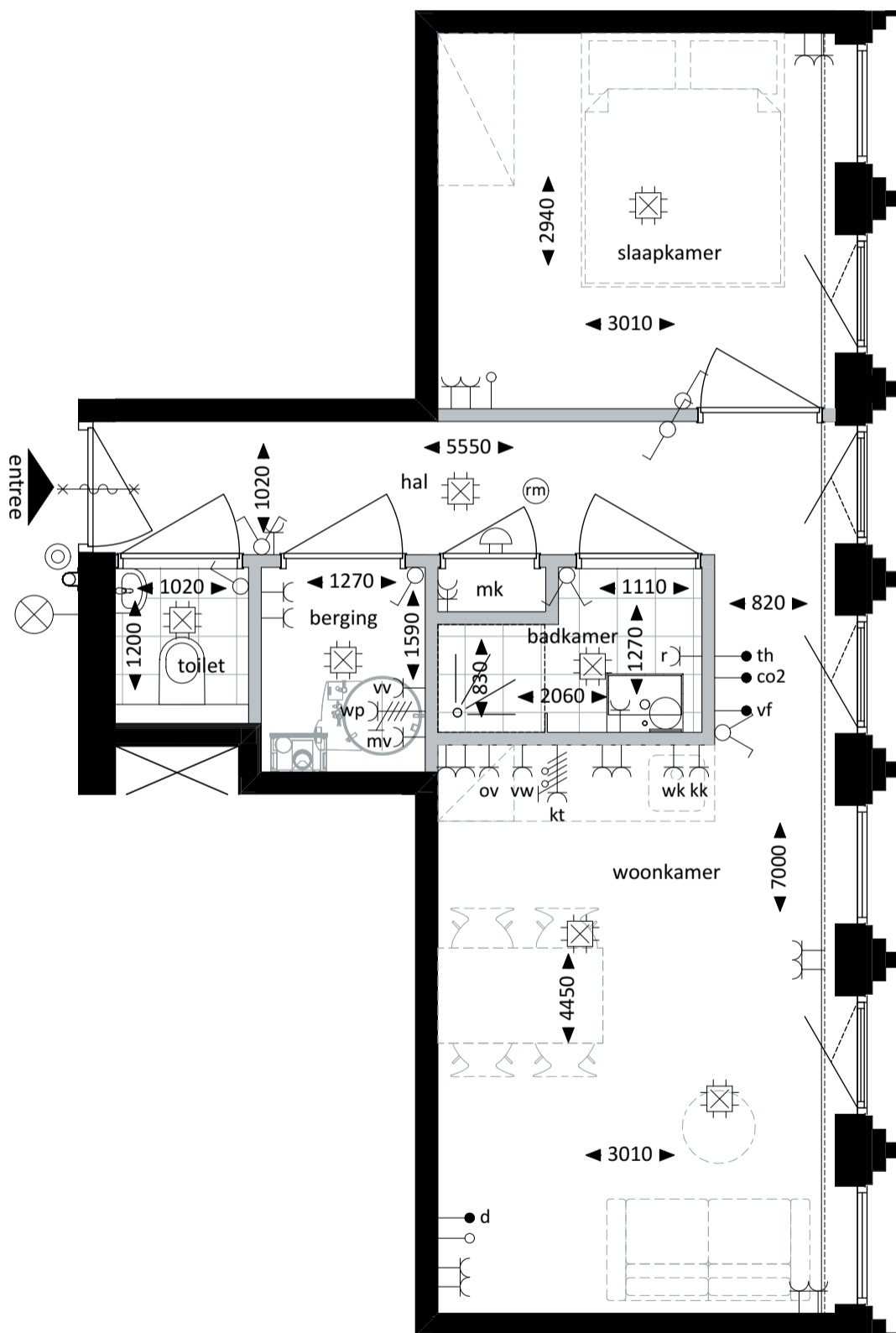
Plattegrond - 1:50
