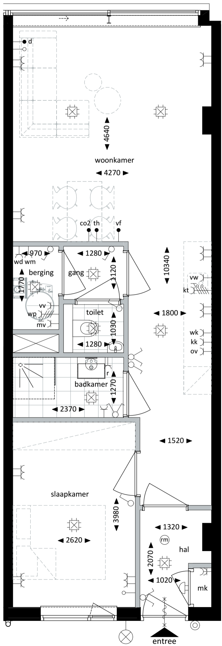
Plattegrond - 1:50
