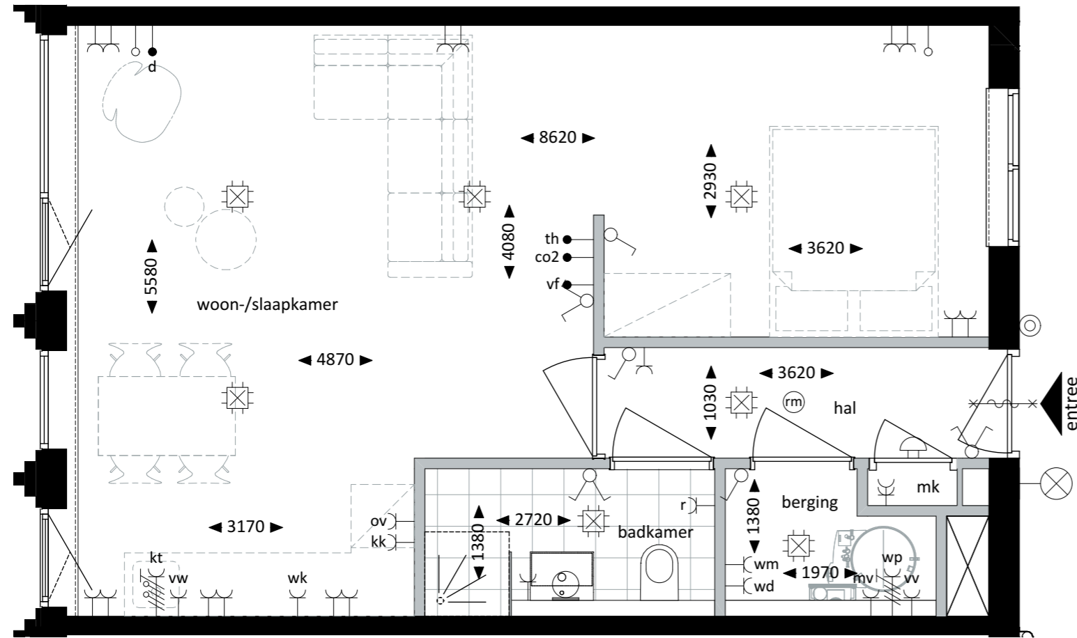
Plattegrond - 1:50
