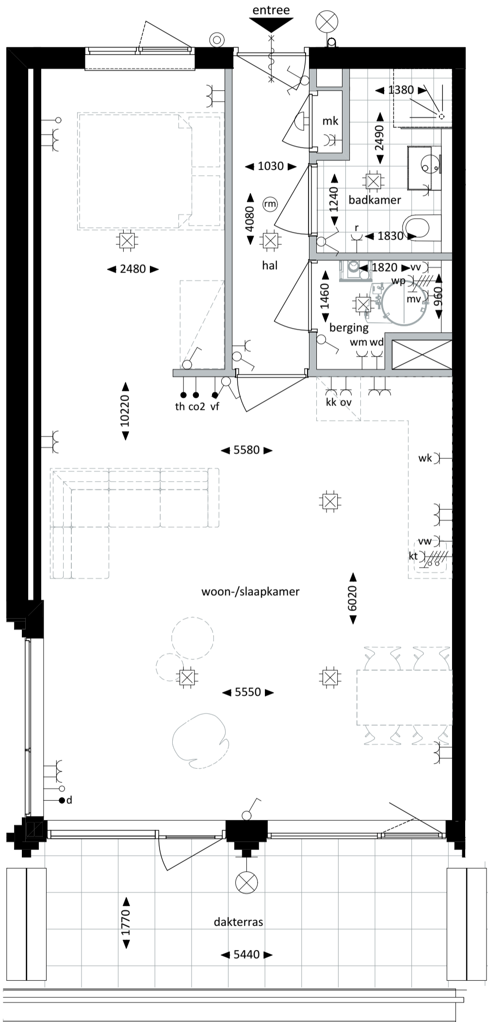
Plattegrond - 1:500
