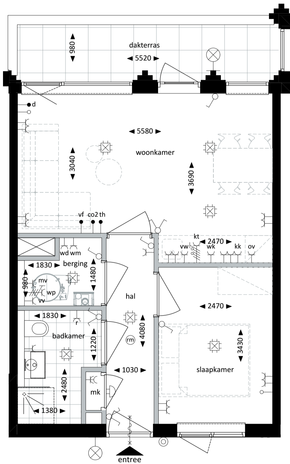
Plattegrond - 1:50
