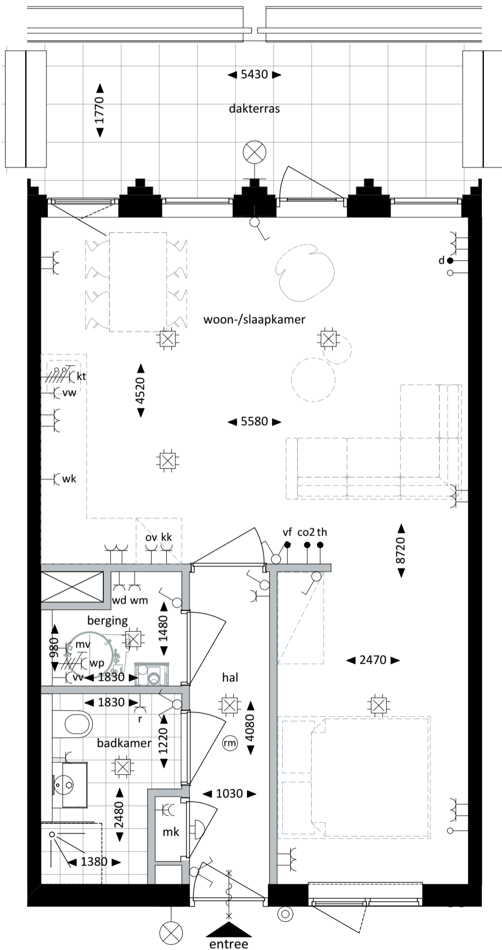
Plattegrond - 1:50
