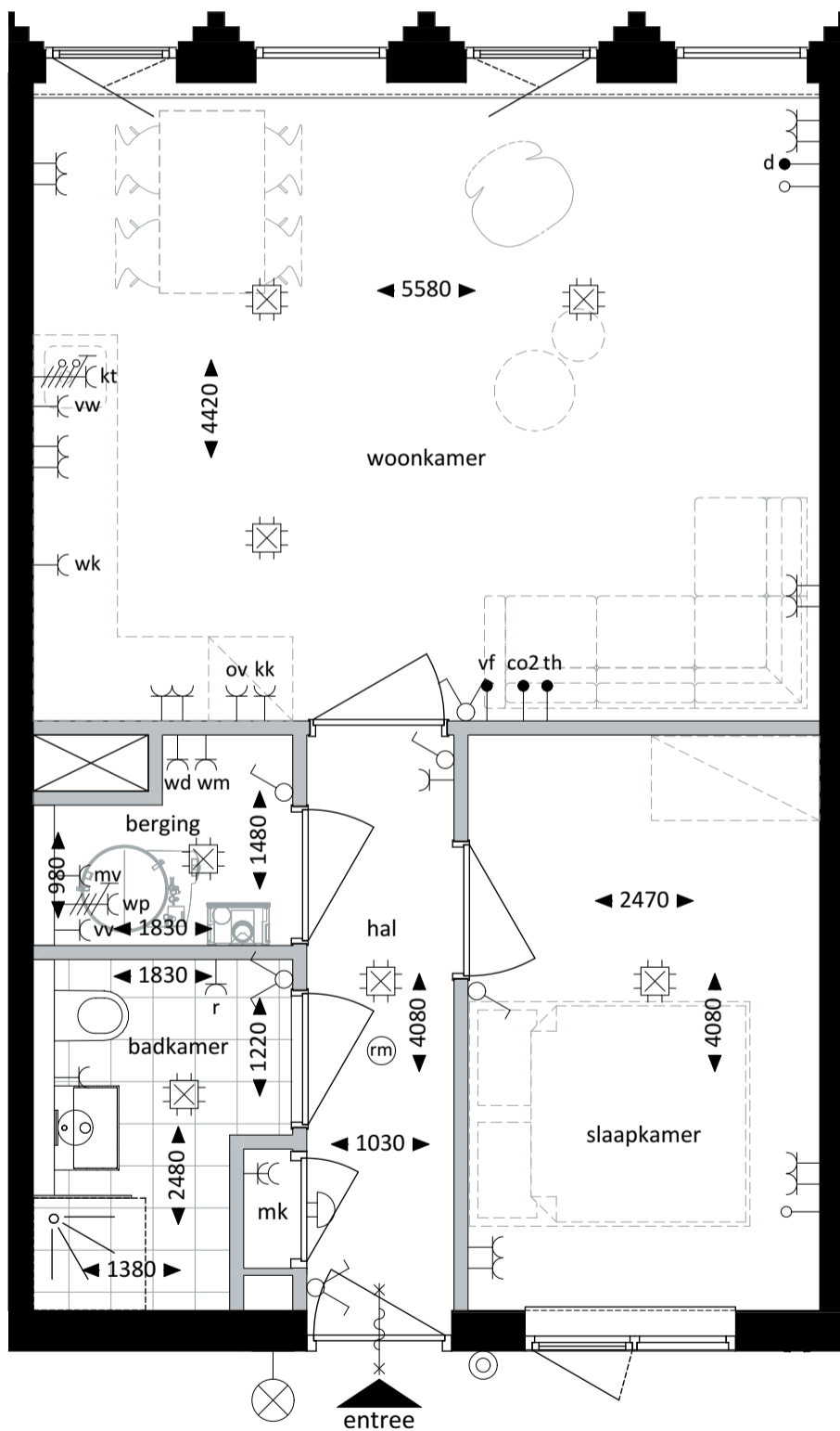
Plattegrond - 1:50
