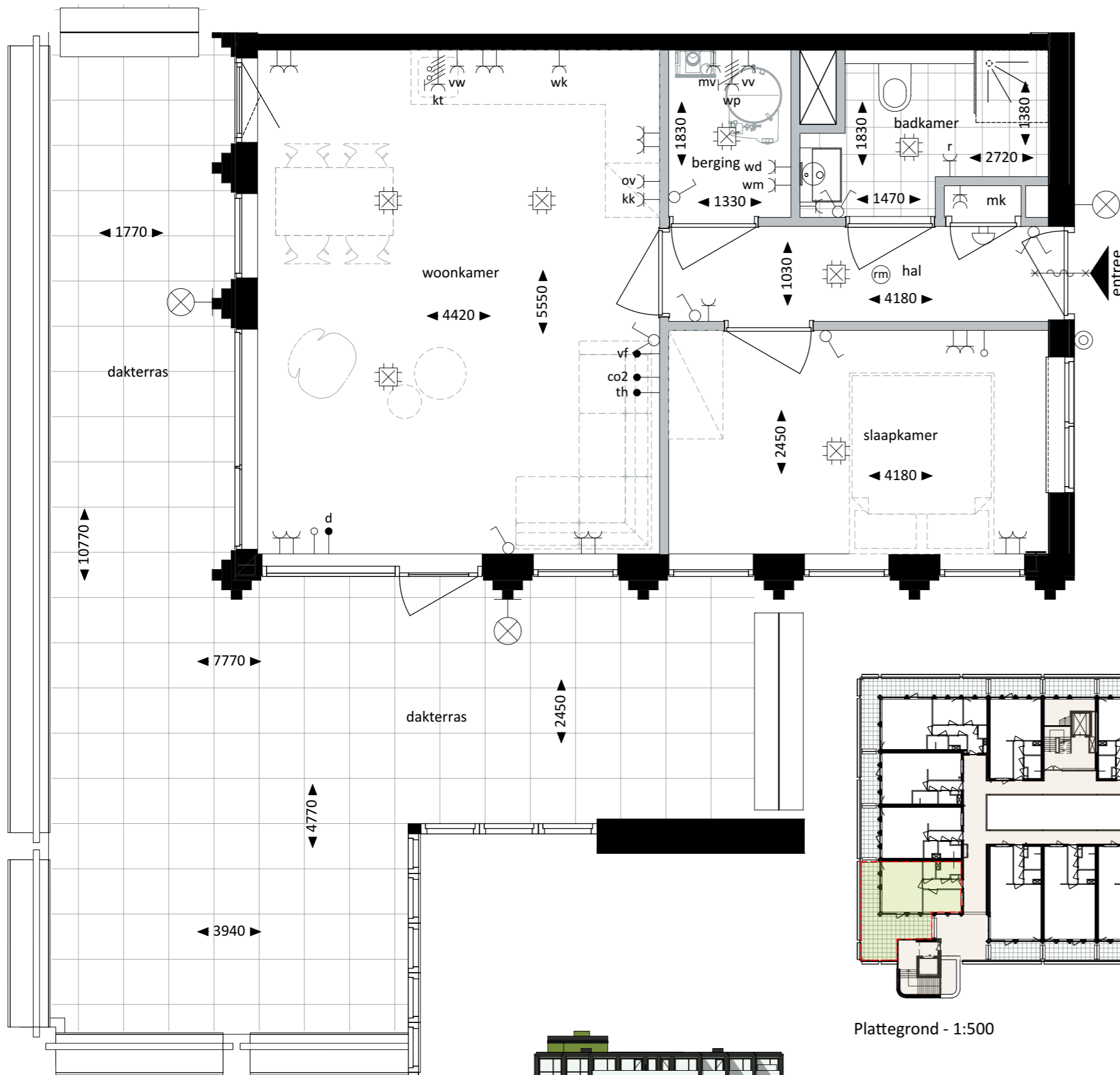
Plattegrond - 1:50
