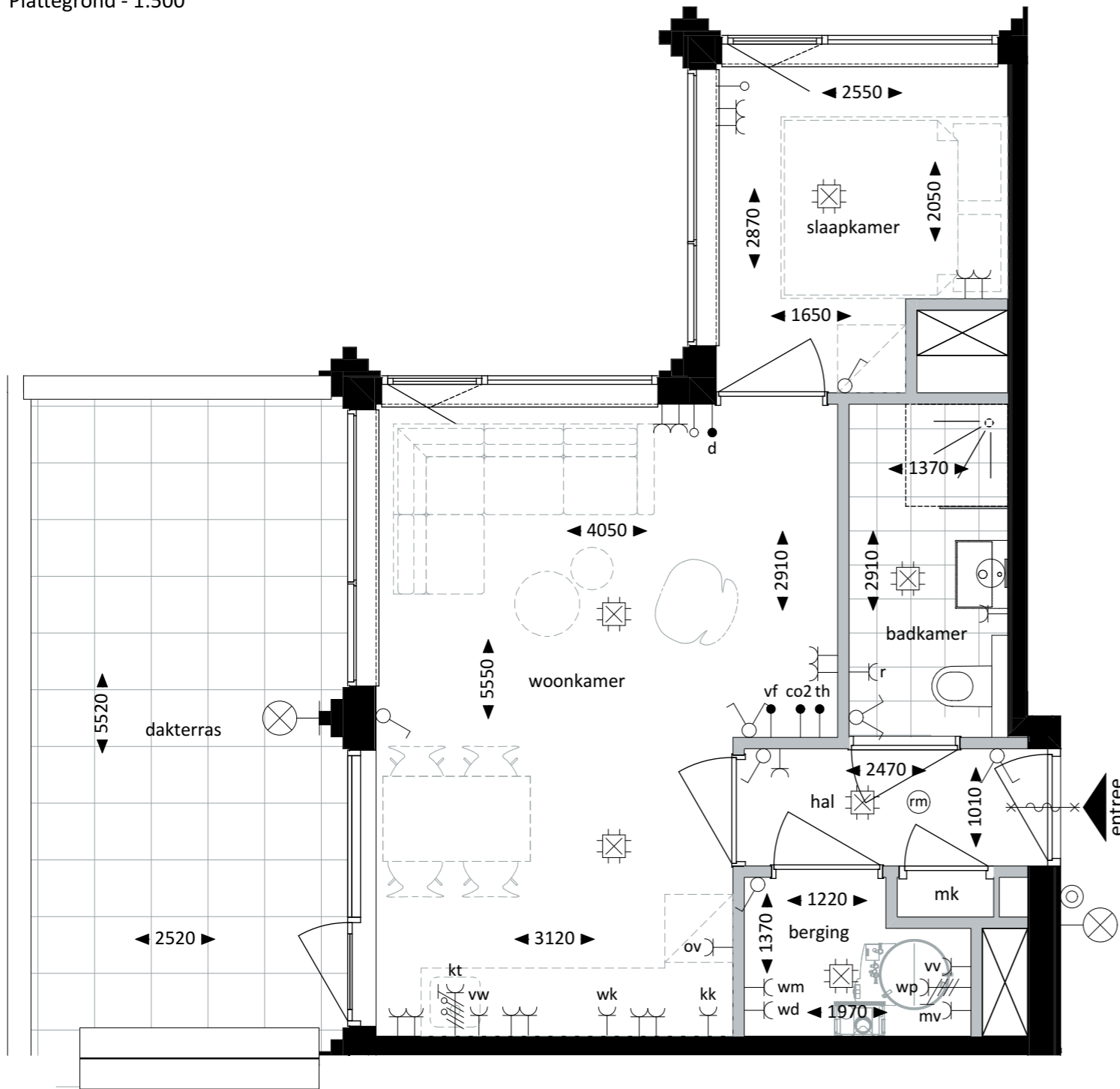
Plattegrond - 1:50
