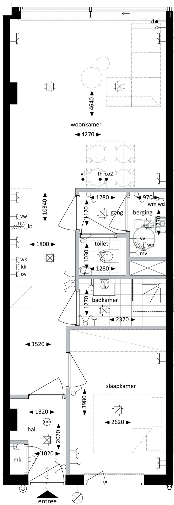
Plattegrond - 1:50
