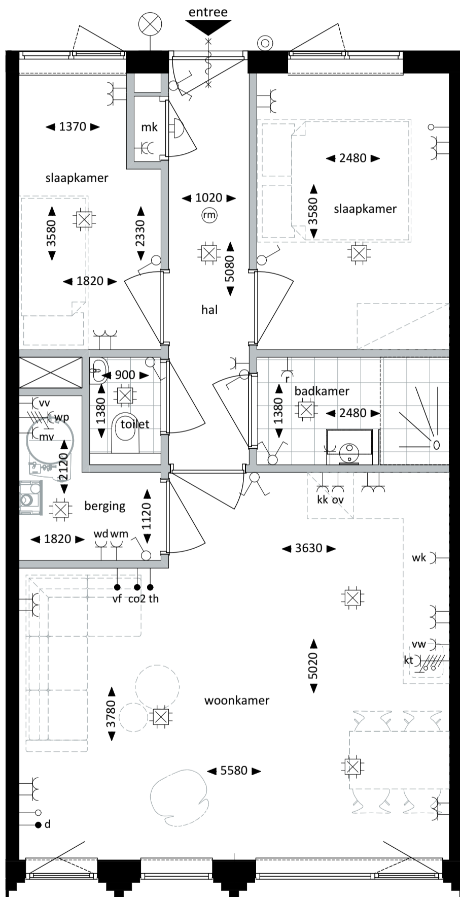
Plattegrond - 1:50
