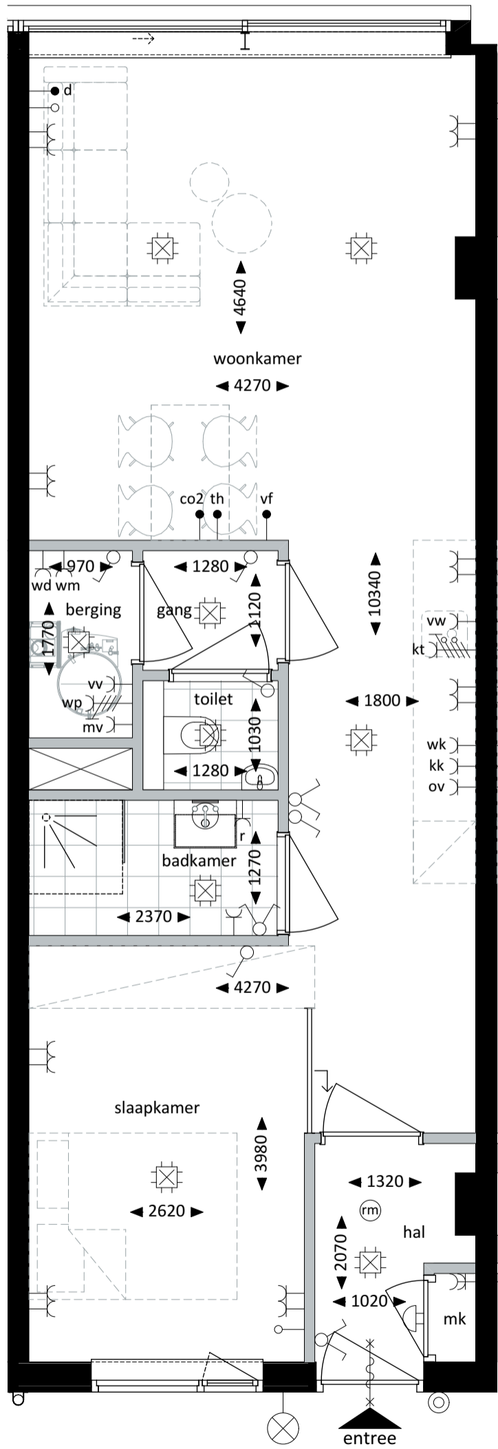
Plattegrond - 1:50
