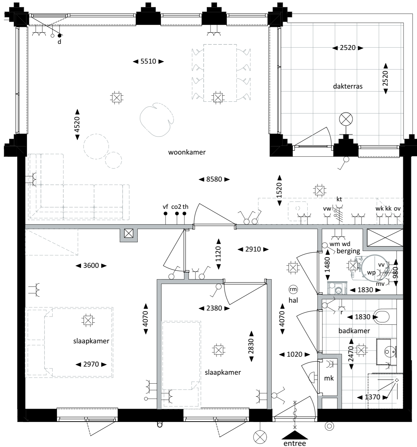
Plattegrond - 1:50
