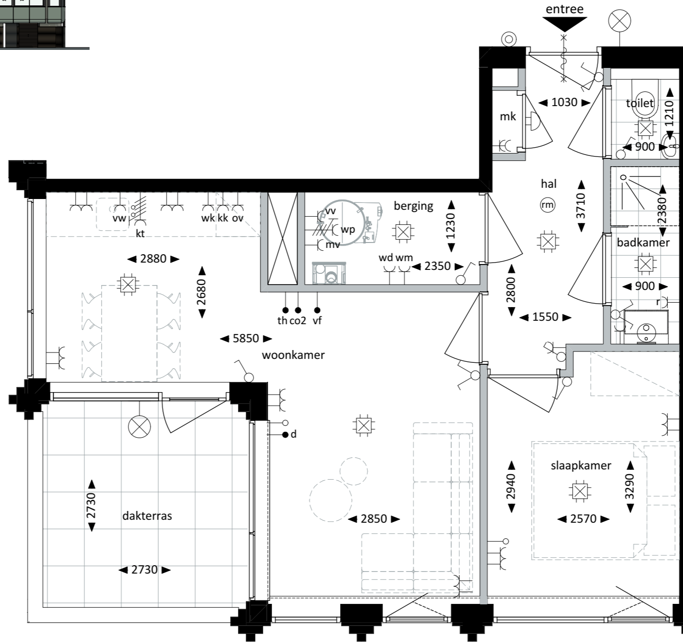
Plattegrond - 1:50
