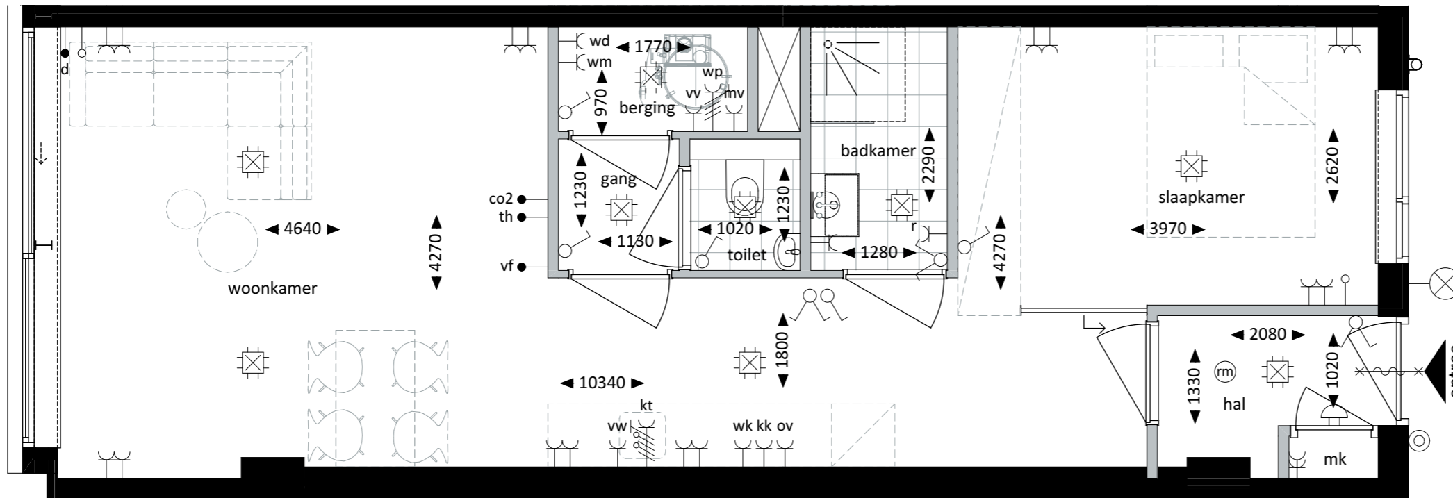
Plattegrond - 1:50
