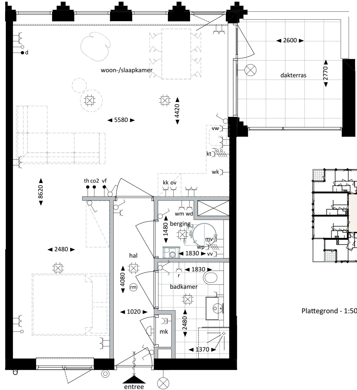
Plattegrond - 1:50
