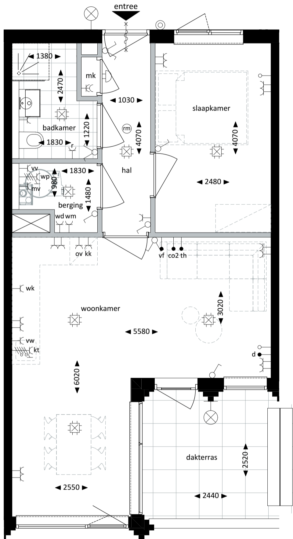
Plattegrond - 1:50
