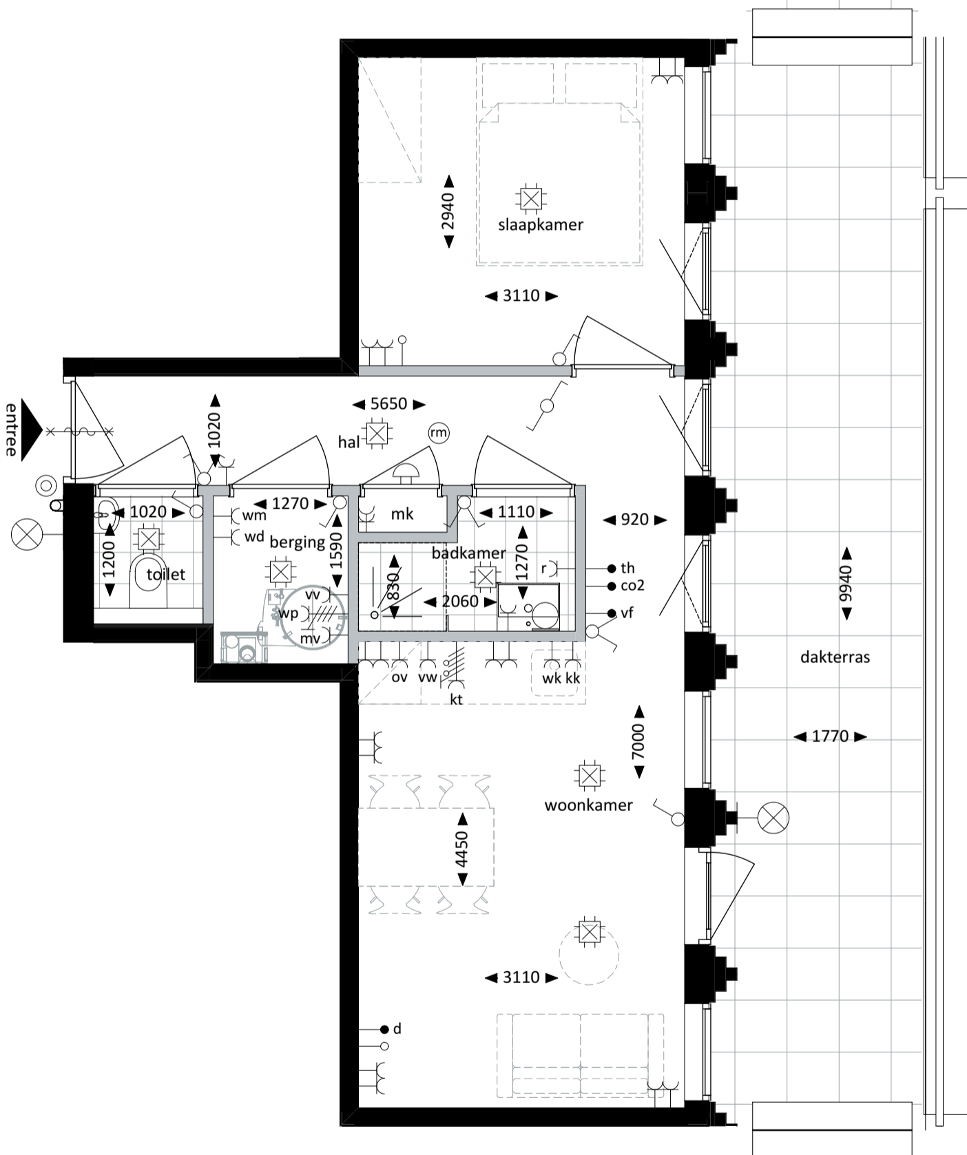
Plattegrond - 1:50
