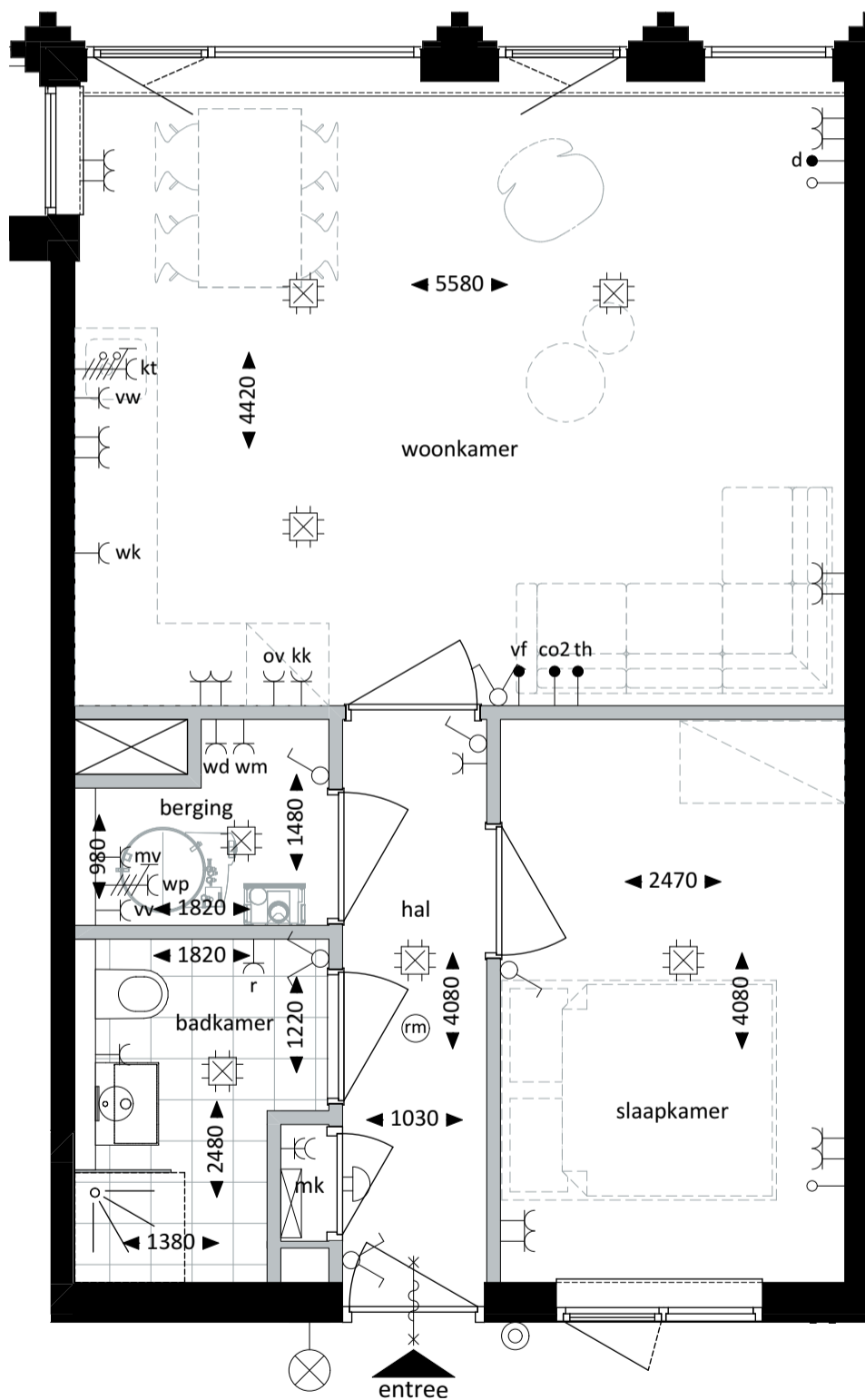
Plattegrond - 1:50
