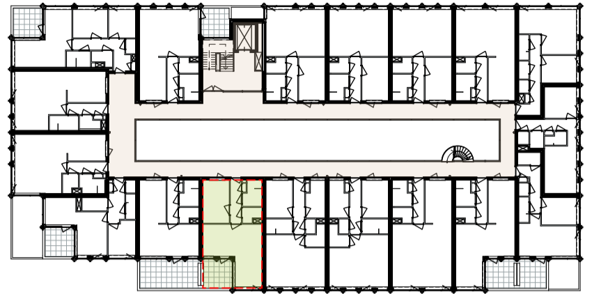
Plattegrond - 1:500
