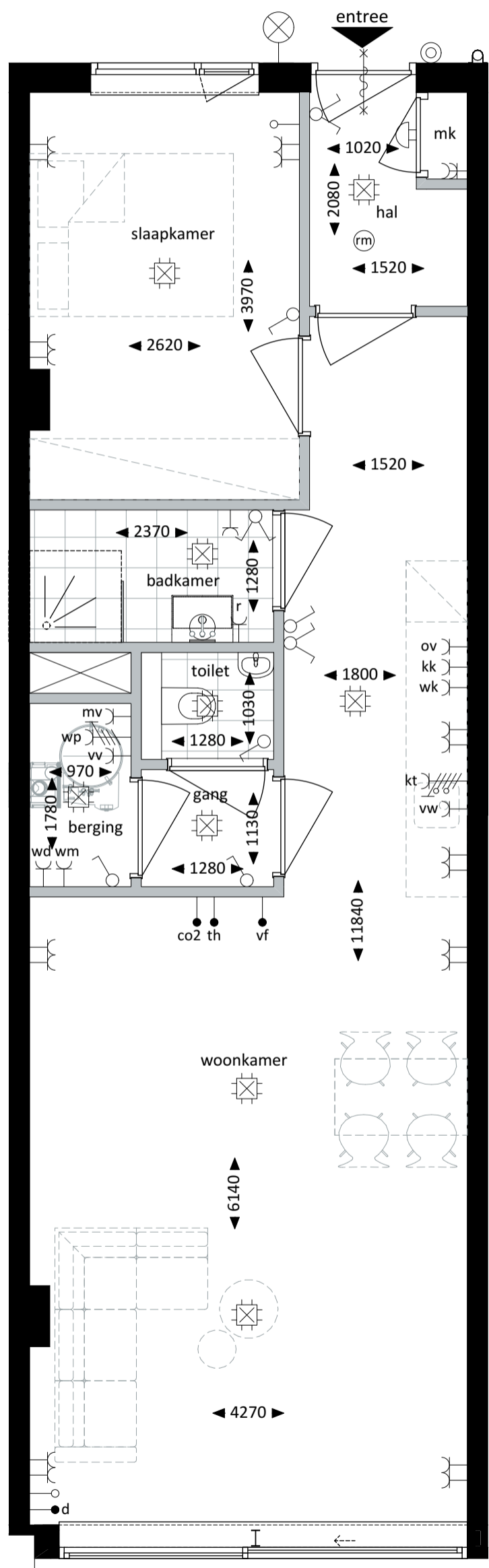
Plattegrond - 1:50
